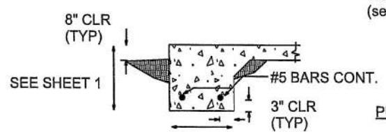
THICKENED EDGE
