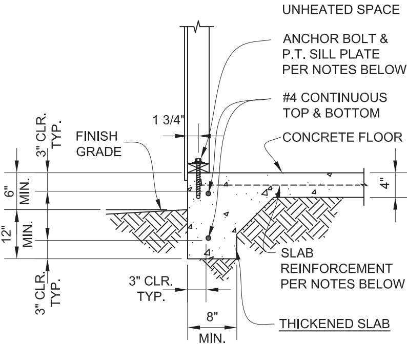
4 CONCRETE FOUNDATION DETAIL SCALE: N.T.S.
