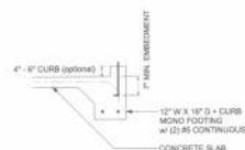
F4 S-2 SCALE: 1/2" = 1'-0"
