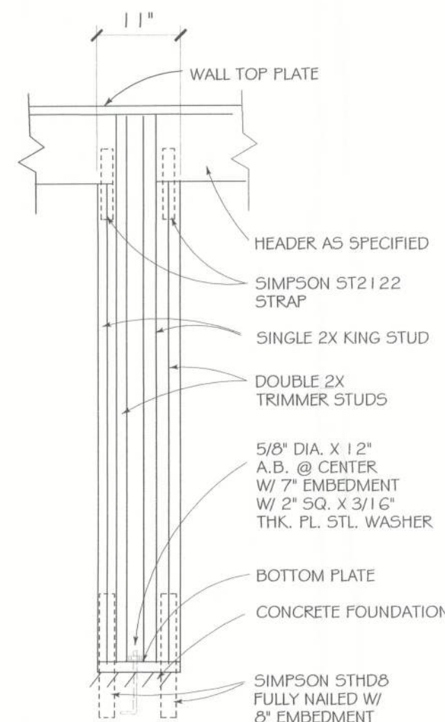
3 GARAGE DOOR SEPARATOR DETAIL
