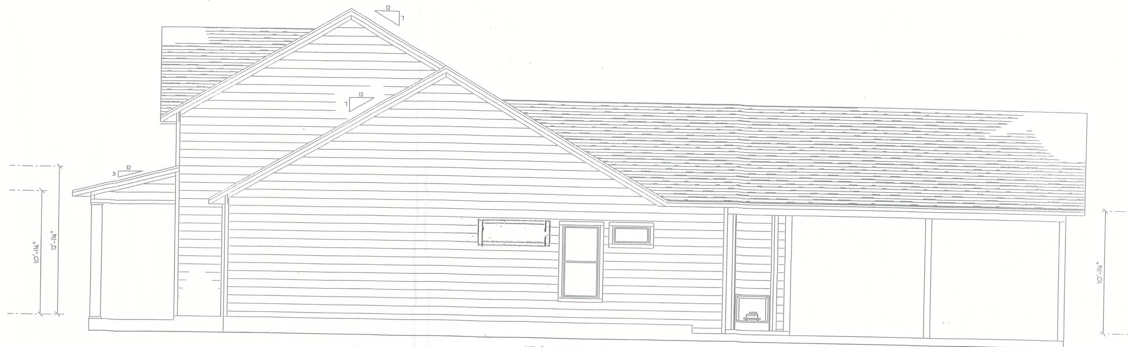
RIGHT ELEVATION
