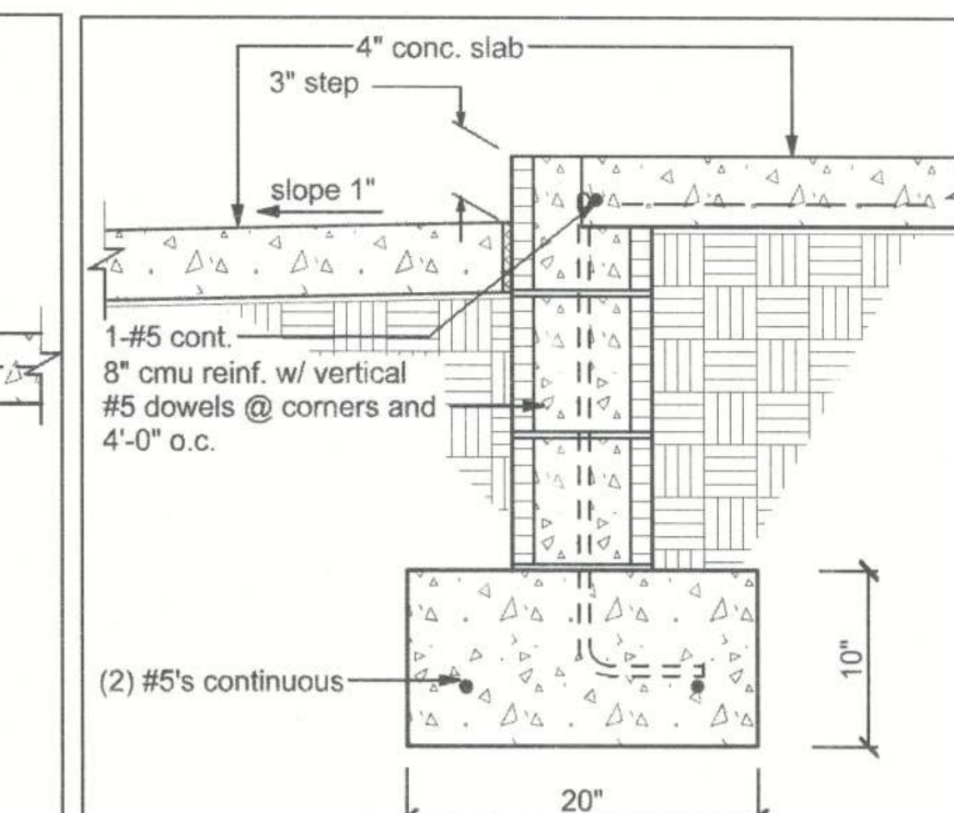
3 STEMWALL SECTION @ PORCH SCALE: 1" = 1'-0"
