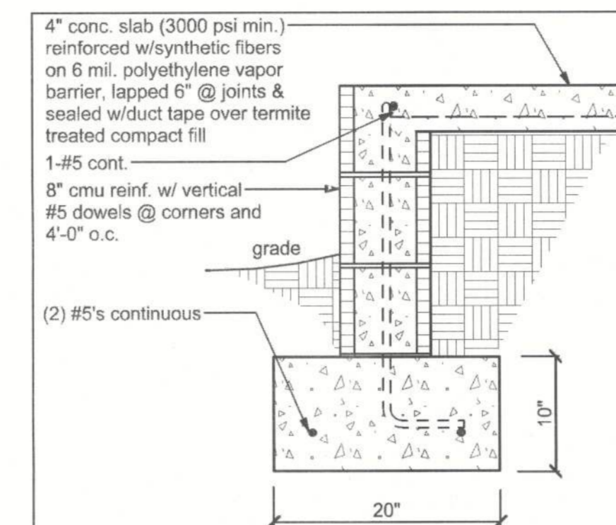
1 STEMWALL SECTION SCALE: 1" = 1'-0"
