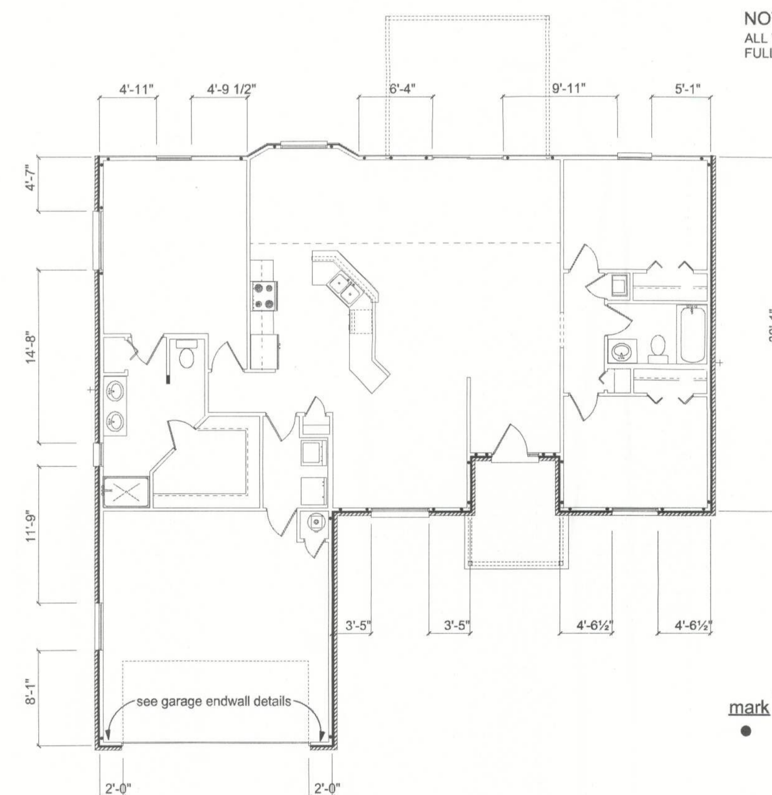
SHEARWALL LAYOUT SCALE: 1/8" = 1'-0"
