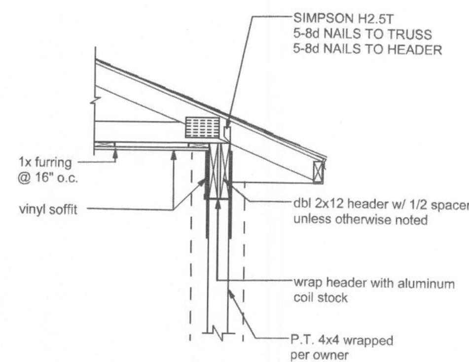
A PORCH SECTION SCALE: 3/4" = 1'-0"
