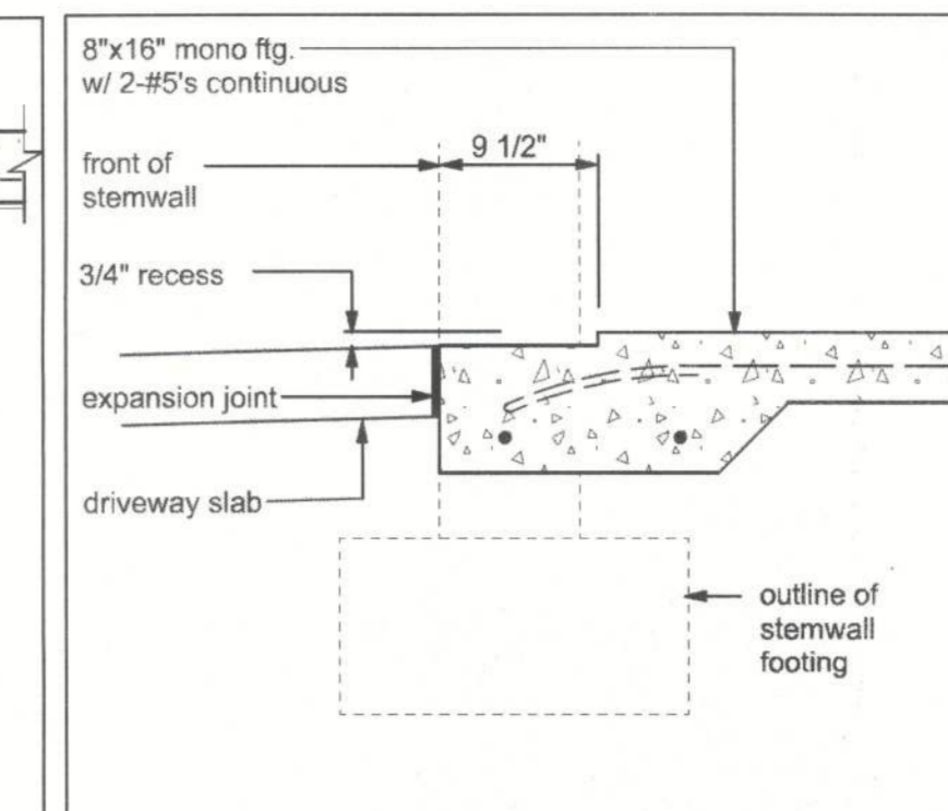
2 FTG. SECTION SCALE: 1" = 1'-0"
