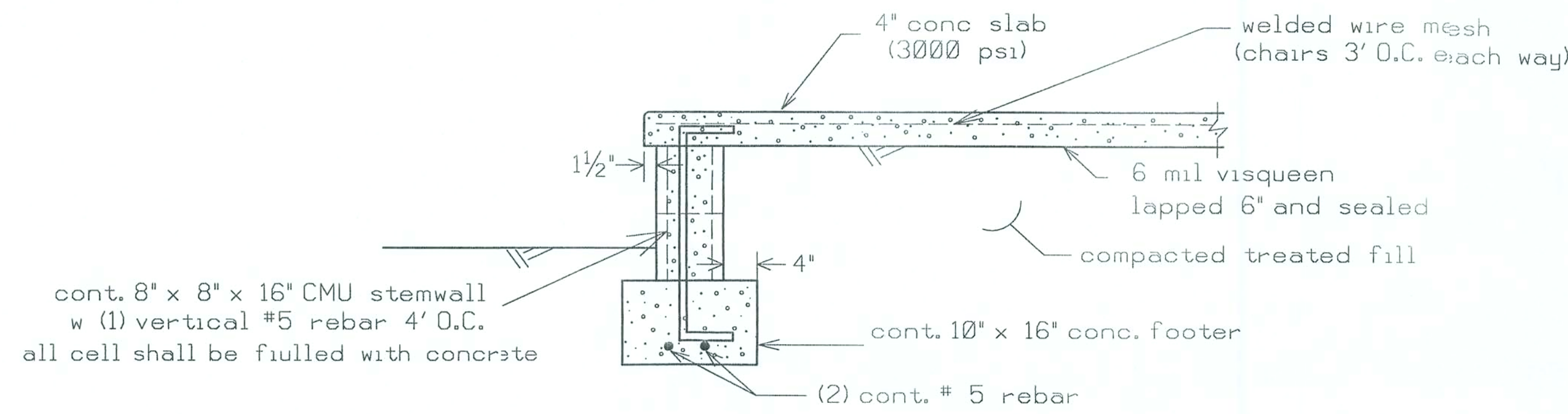
PORCH FOUNDATION(N.T.S.)
