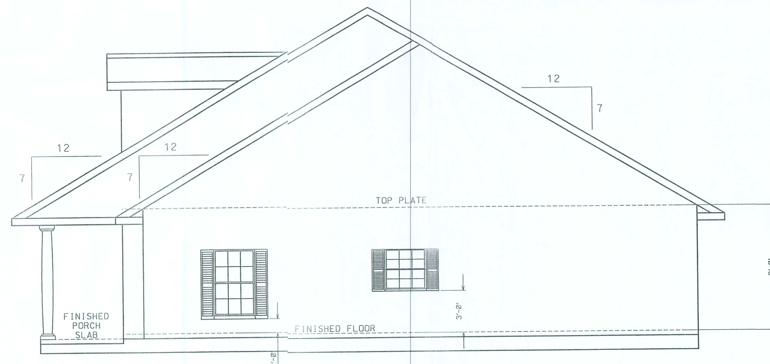
RIGHT ELEVATION
