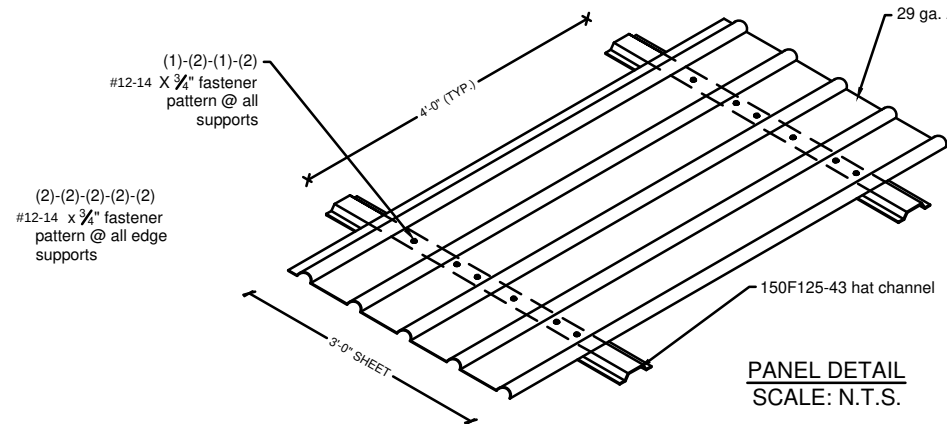
PANEL DETAIL SCALE: N.T.S.
