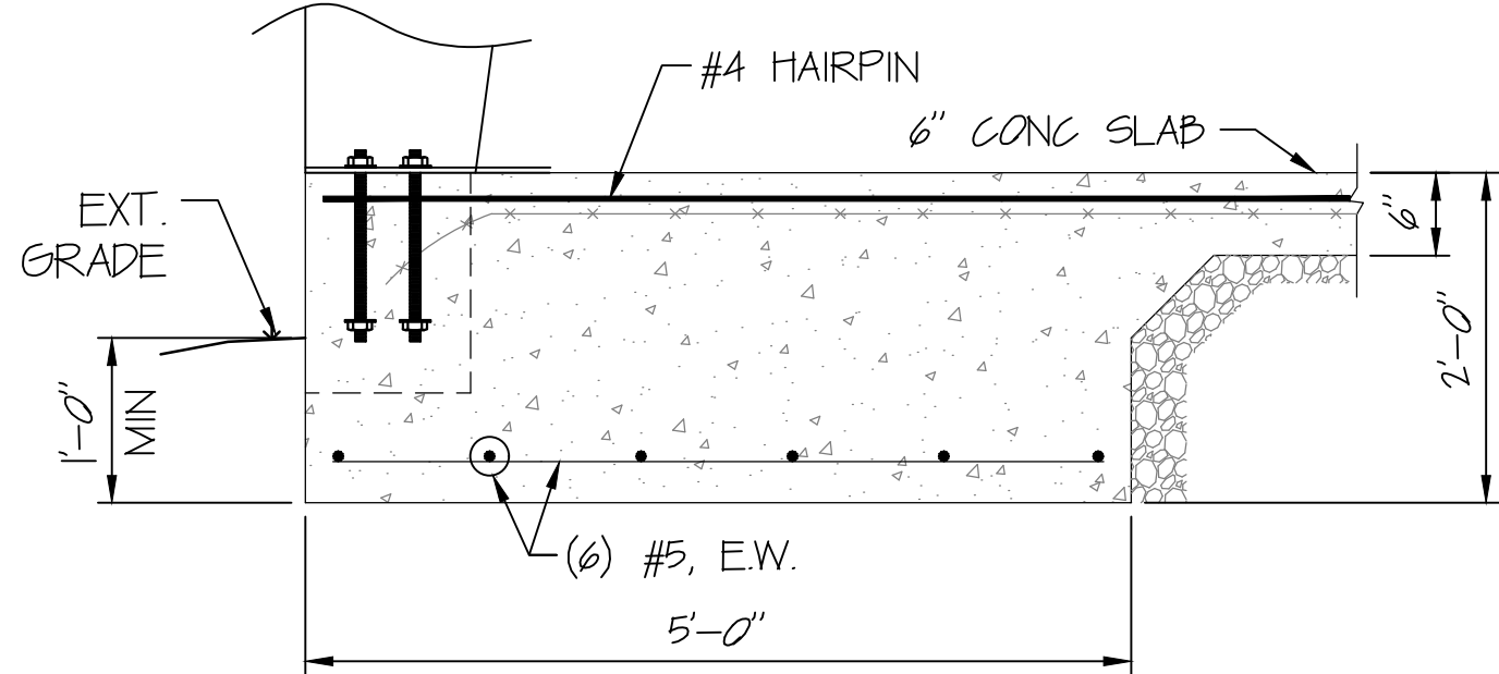
SECTION 5 N.T.S.
