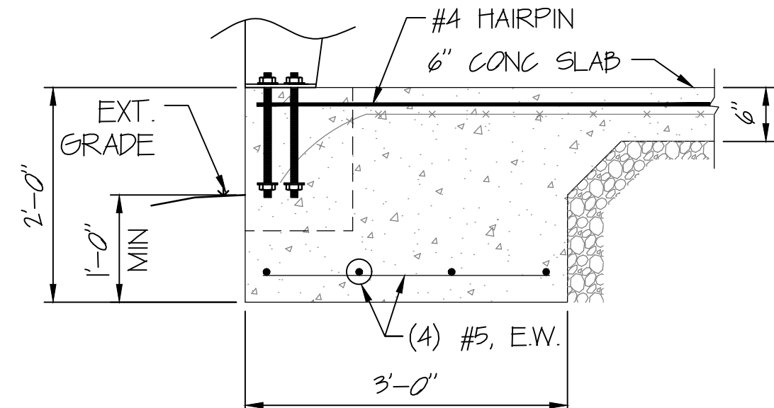
SECTION 3 N.T.S.
