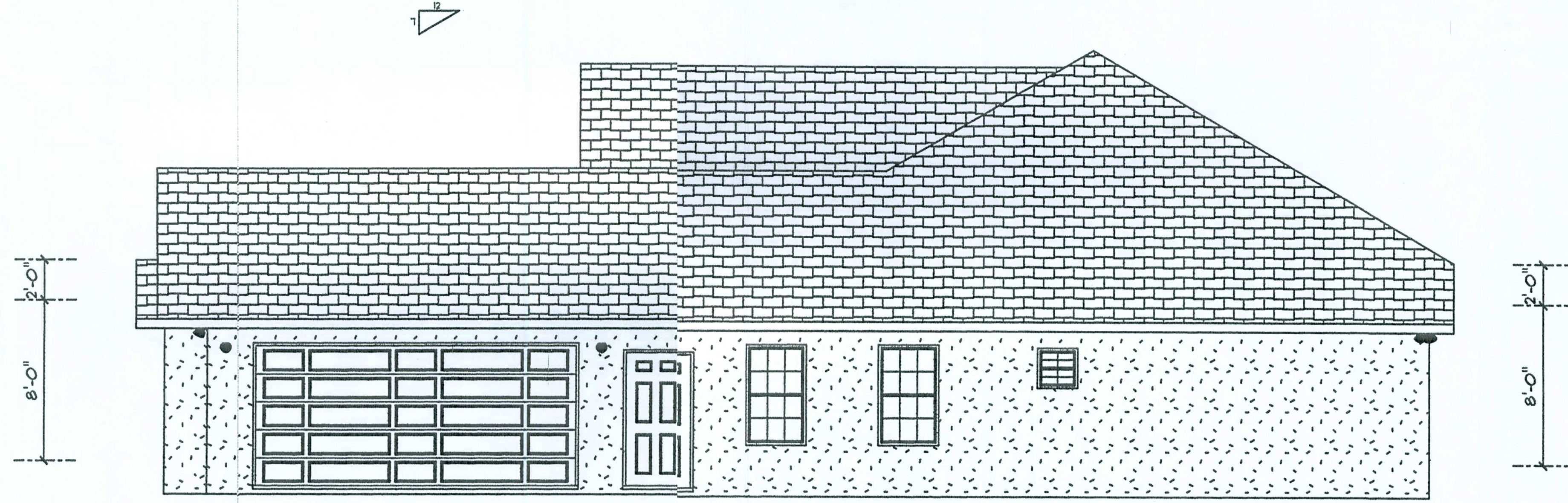
RIGHT ELEVATION
