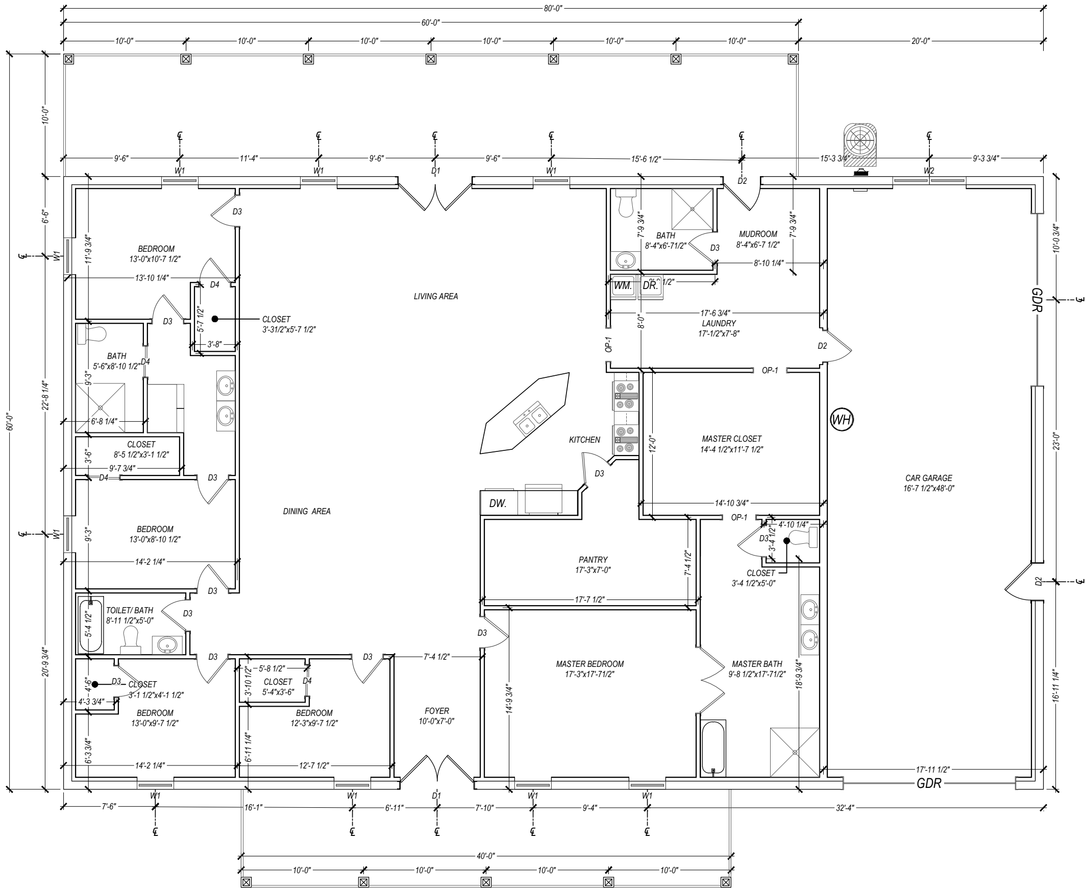
1 FLOOR PLAN A-100 SCALE: 1/8" = 1'
