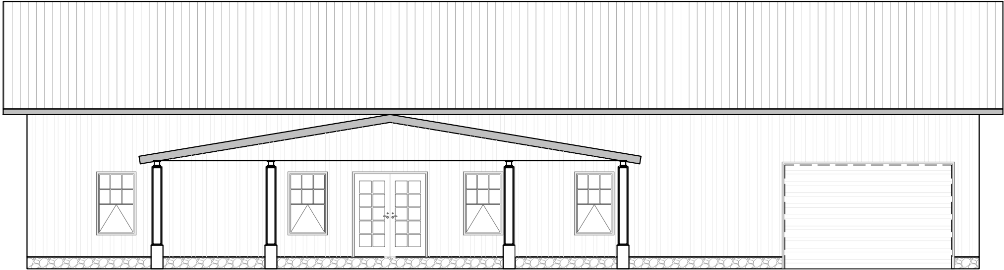
1 A-200 ELEVATION-I SCALE: 1/8" = 1'
