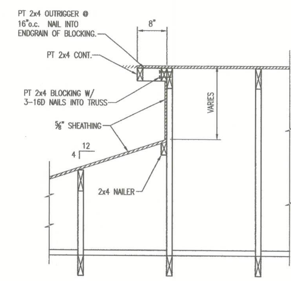
SECTION C SCALE: 3/8" = 1'-0"
