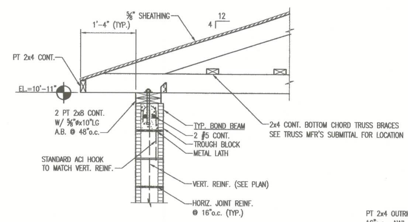
SECTION A SCALE: 3/8" = 1'-0"
