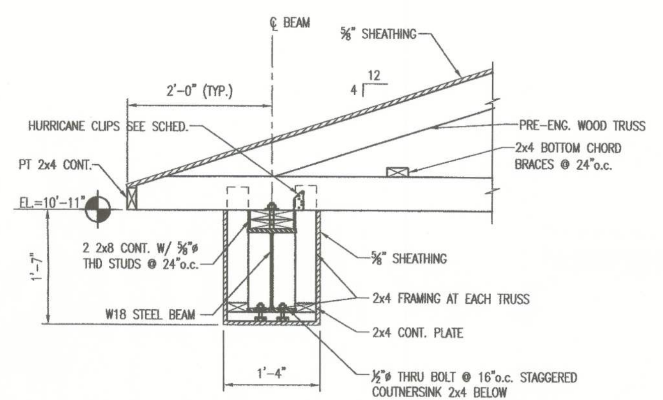
SECTION B SCALE: 3/8" = 1'-0"
