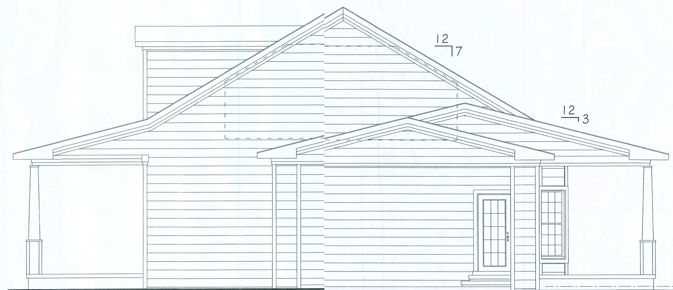
Right Elevation
