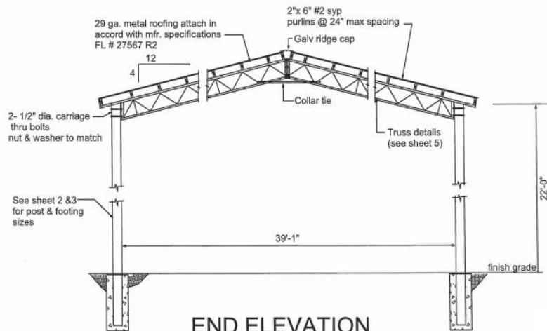
END ELEVATION
