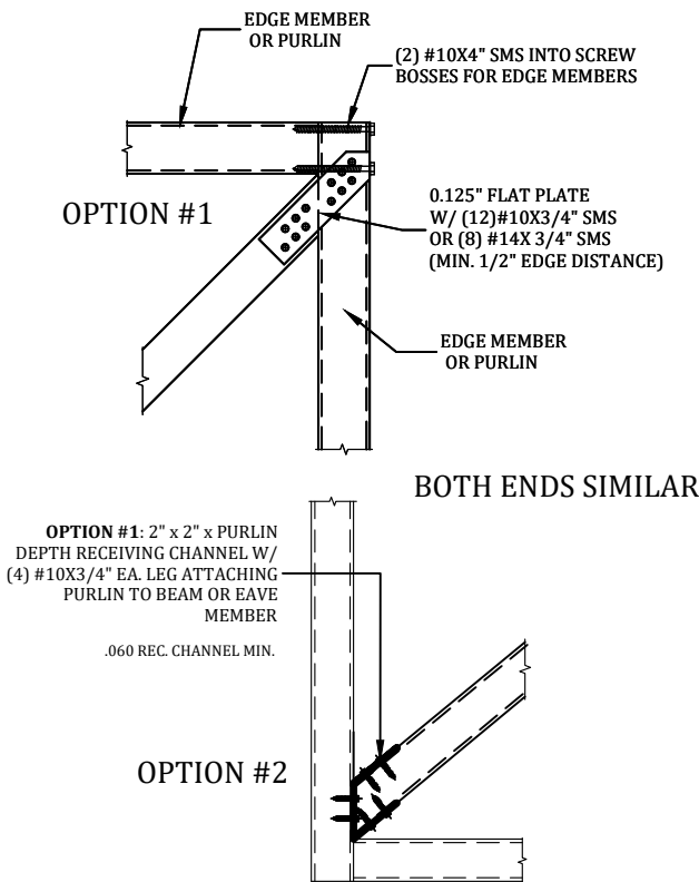
E S-3 ROOF BRACING CONNECTION DETAIL SCALE: N.T.S.
