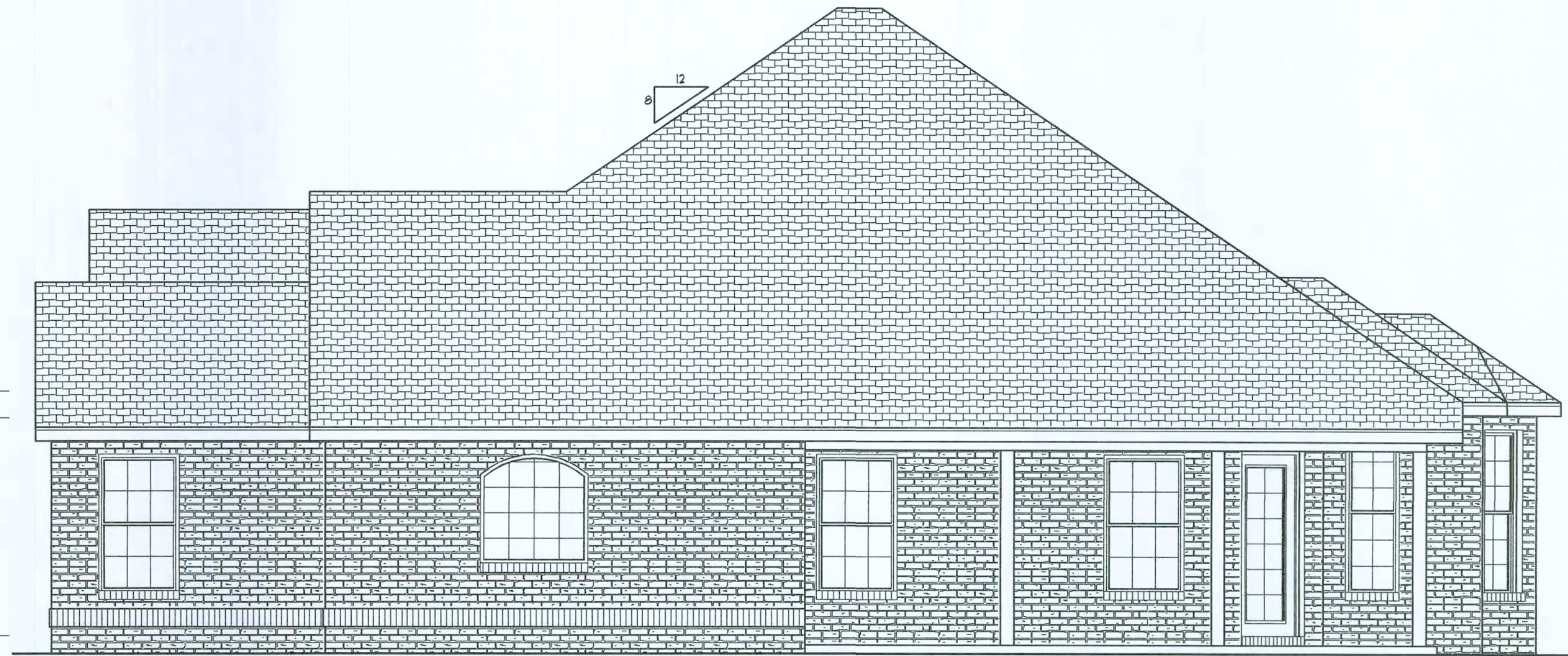
RIGHT ELEVATION
