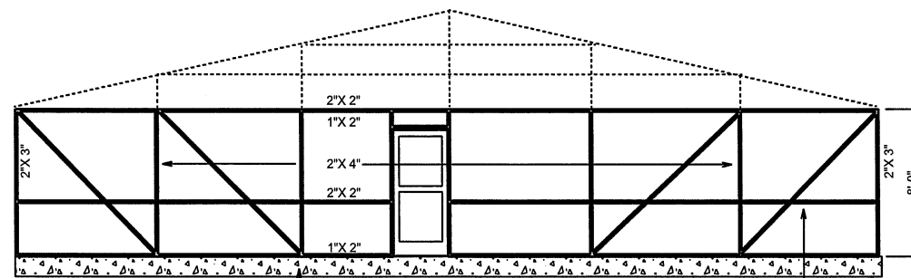
ELEVATION
