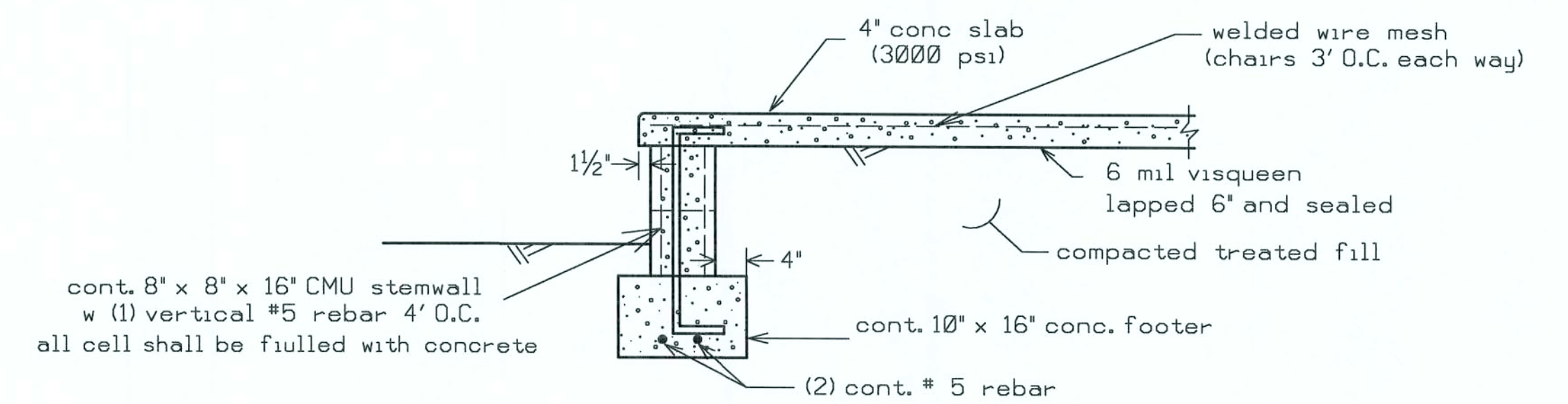
PORCH FOUNDATION (N.T.S.)
