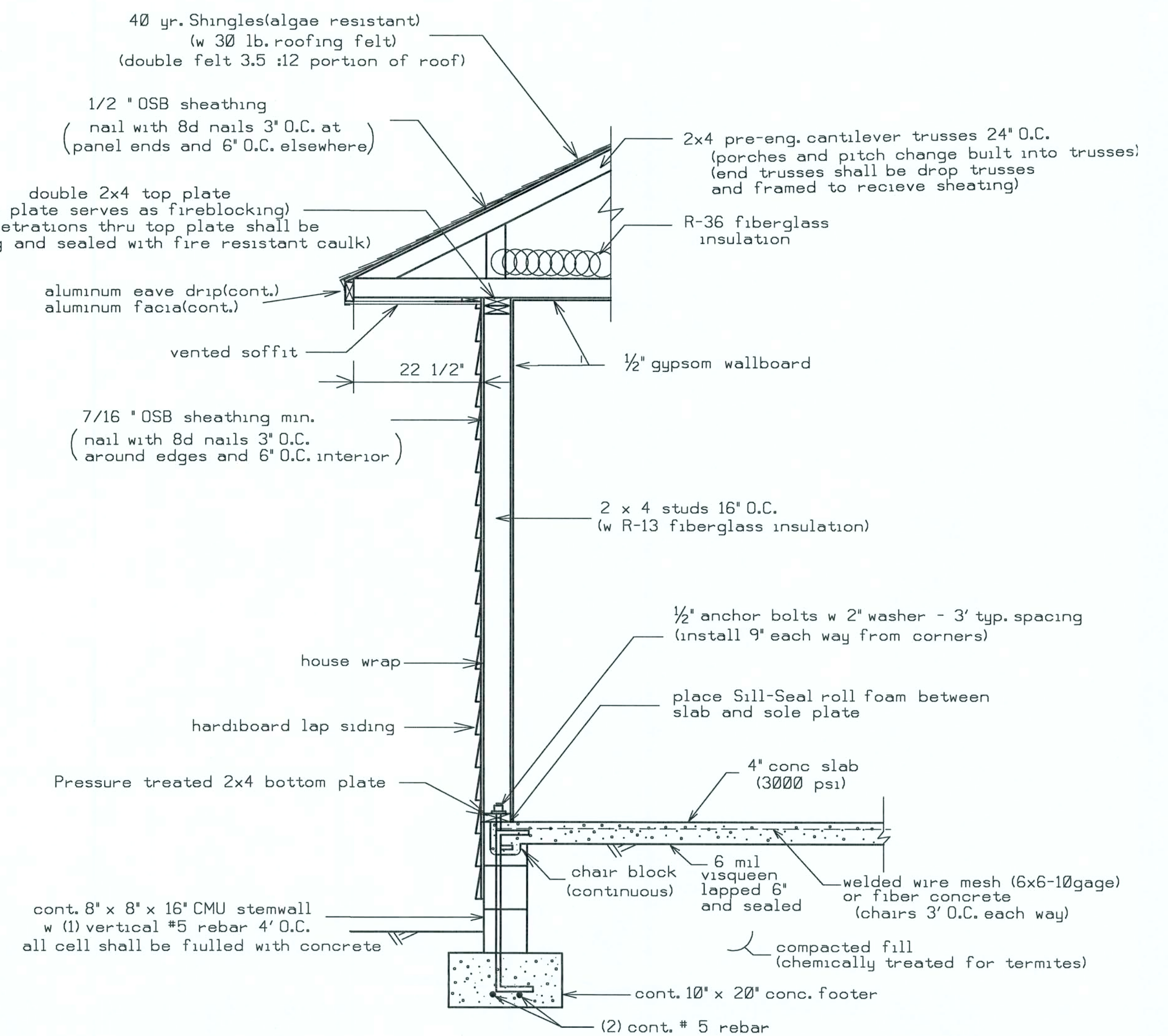
FOOTER DESIGN 1000 PSF WALL DETAIL(TYP.) (N.T.S.)
