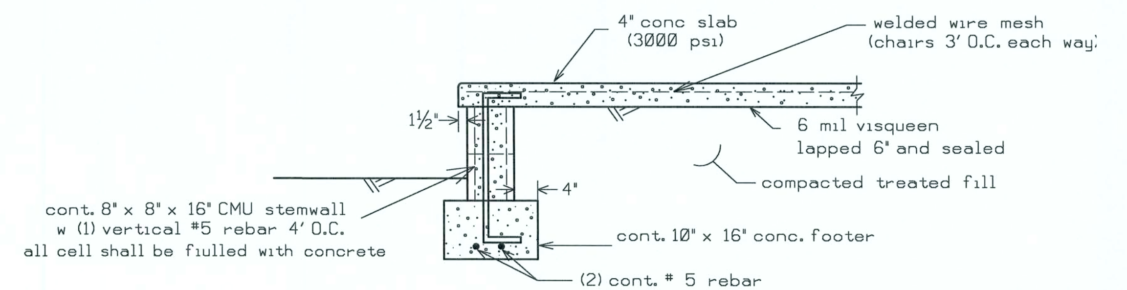
PORCH FOUNDATION (N.T.S.)
