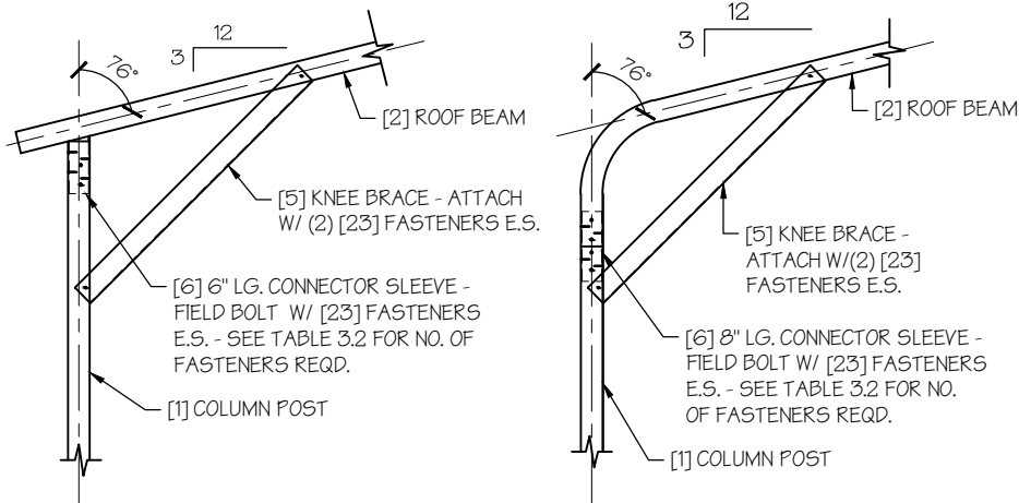
□ A. 'A'-FRAME
