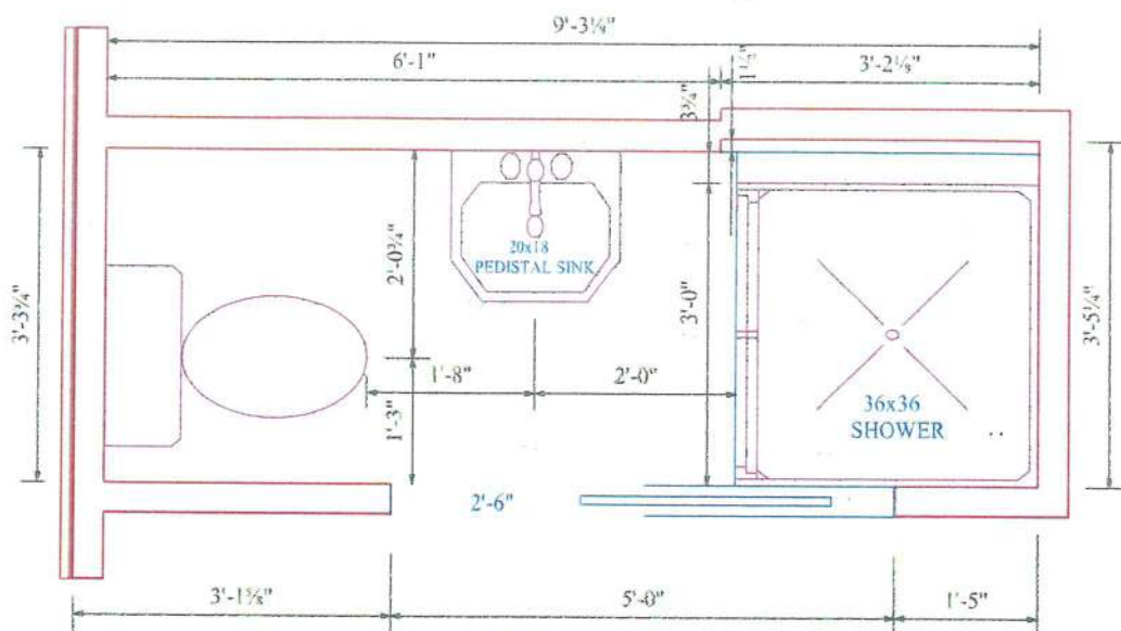
OPTION #1 SCALE: \frac{1}{2}" = 1'-0"
