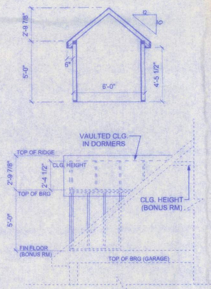
DORMER DETAILS SCALE: 1/4" = 1'-0"
