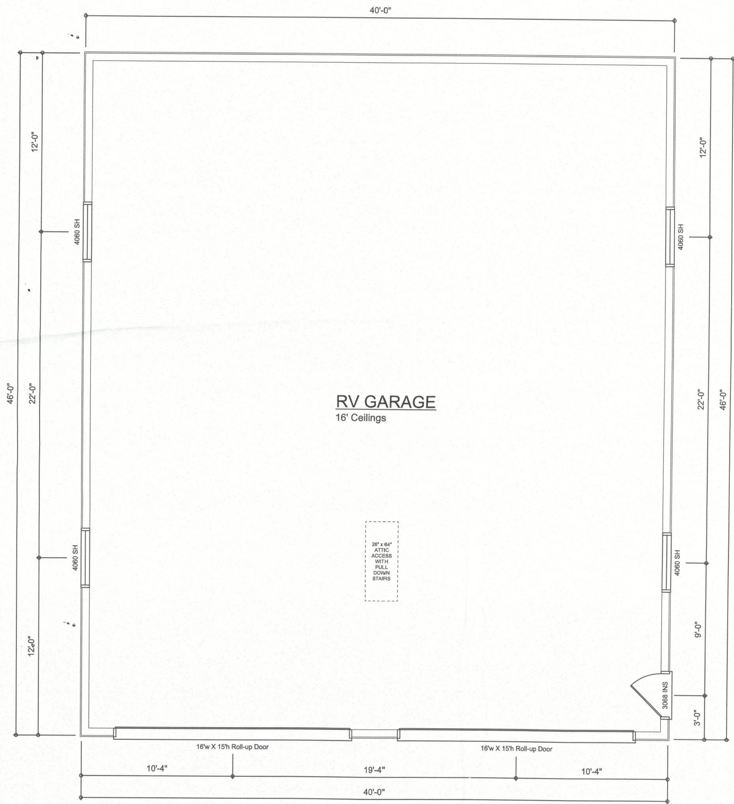
DIMENSIONED PLAN SCALE: 1/4" = 1'-0"
