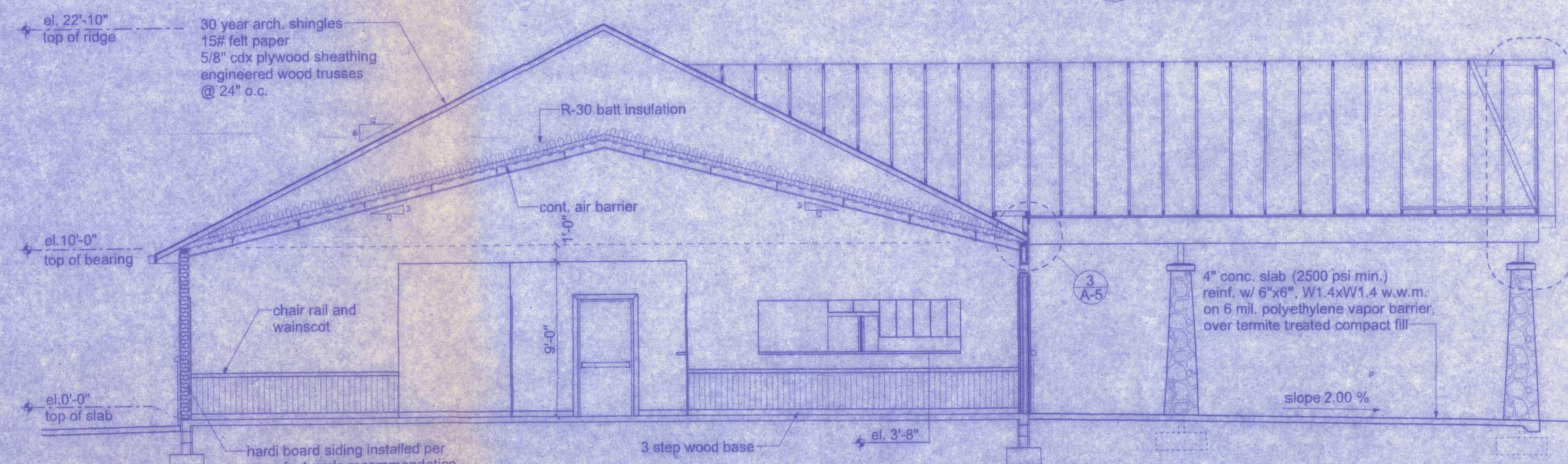
SECTION SCALE: 3/16" = 1'-0"
