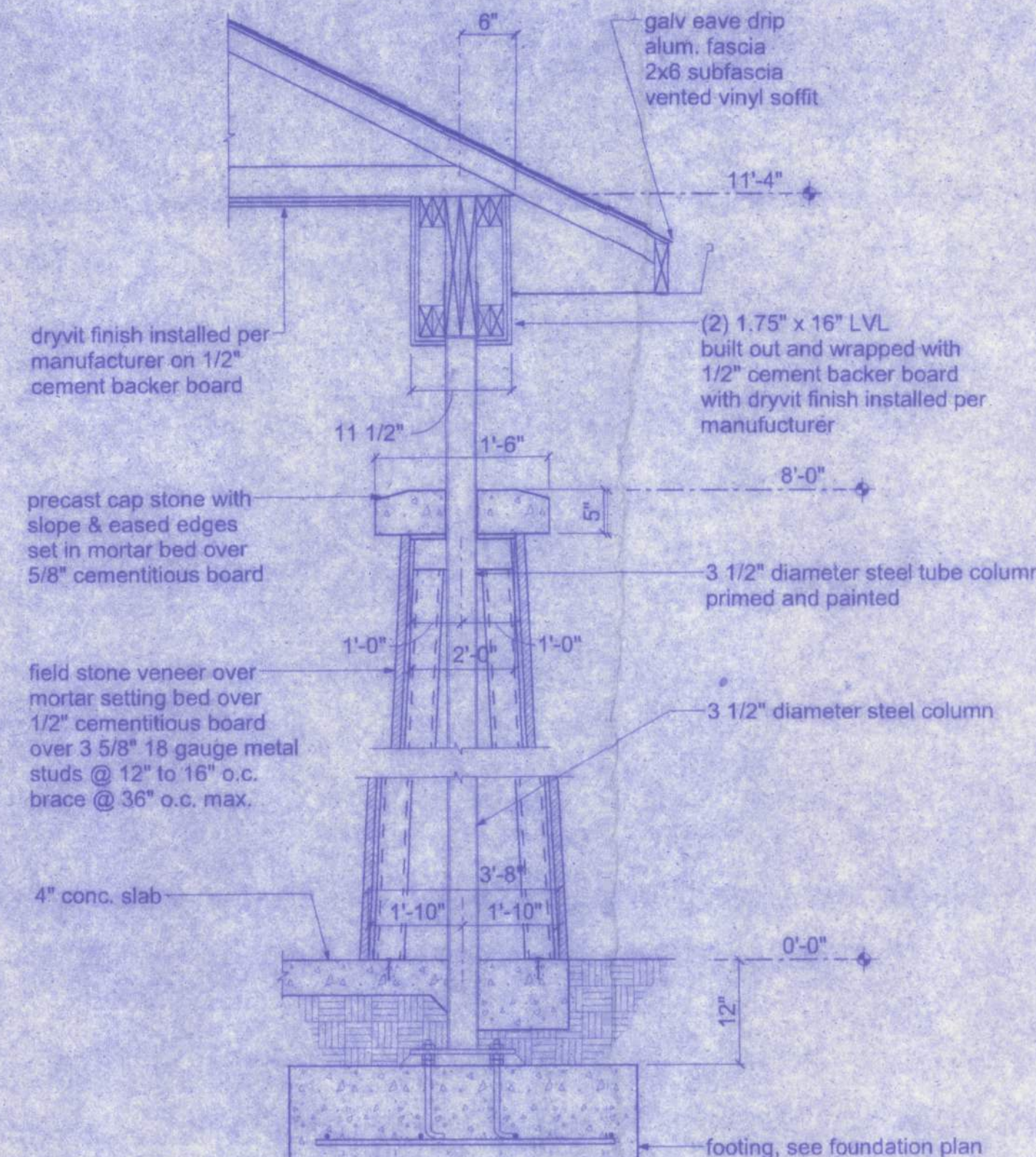
SECTION SCALE: 3/4" = 1'-0"
