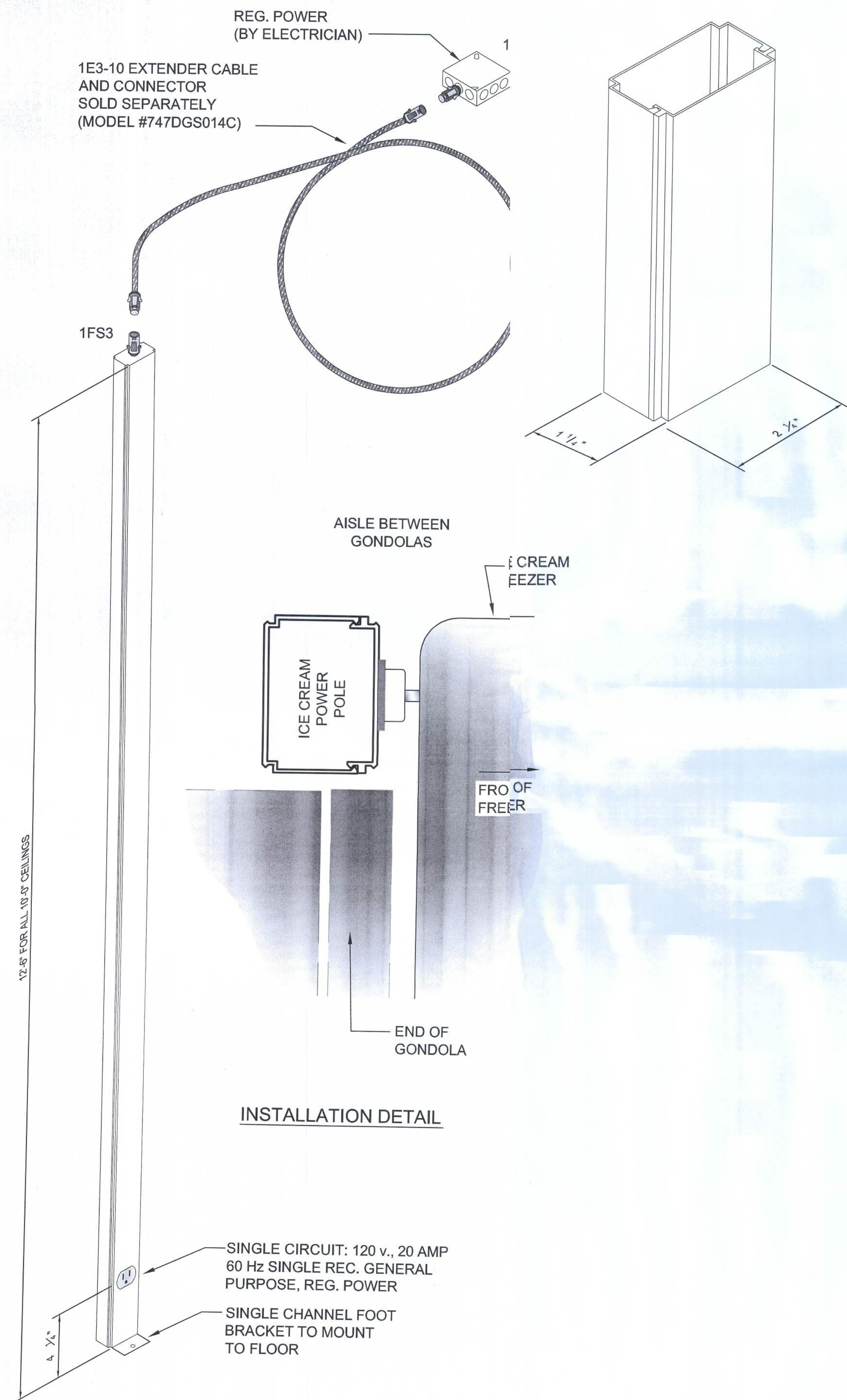
1 747DGS012-12' POWER POLE E3.1.C N.T.S.
