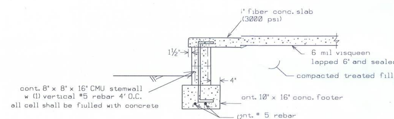
PORCH FOUNDATIO (N.T.S.)
