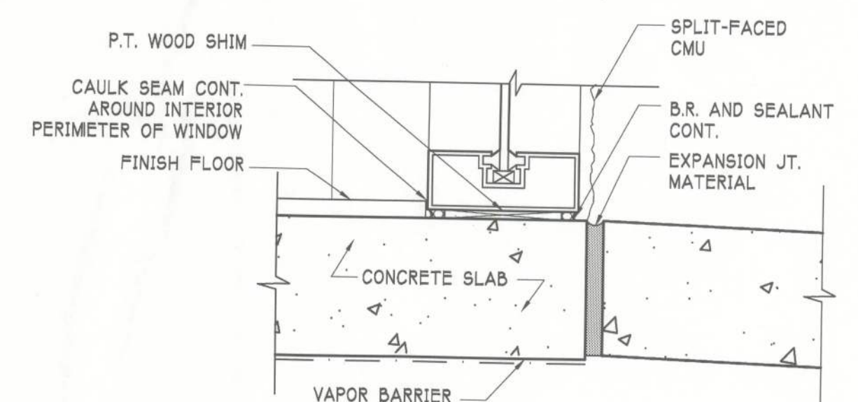
EXT. STOREFRONT SILL
