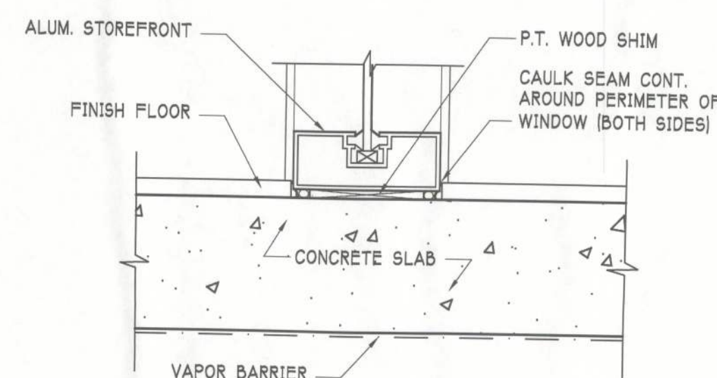
INT. STOREFRONT SILL
