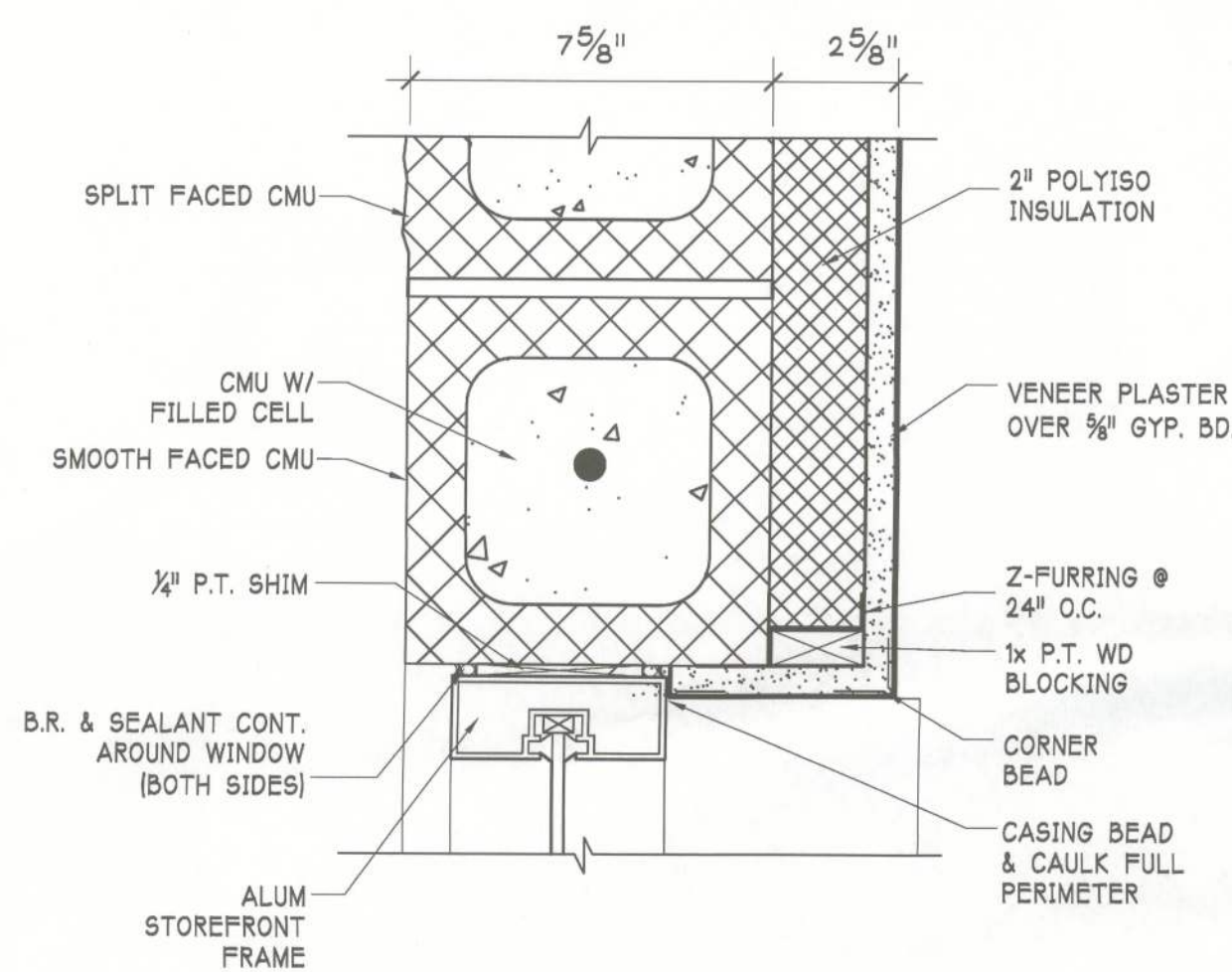
WINDOW JAMB / CMU WALL
