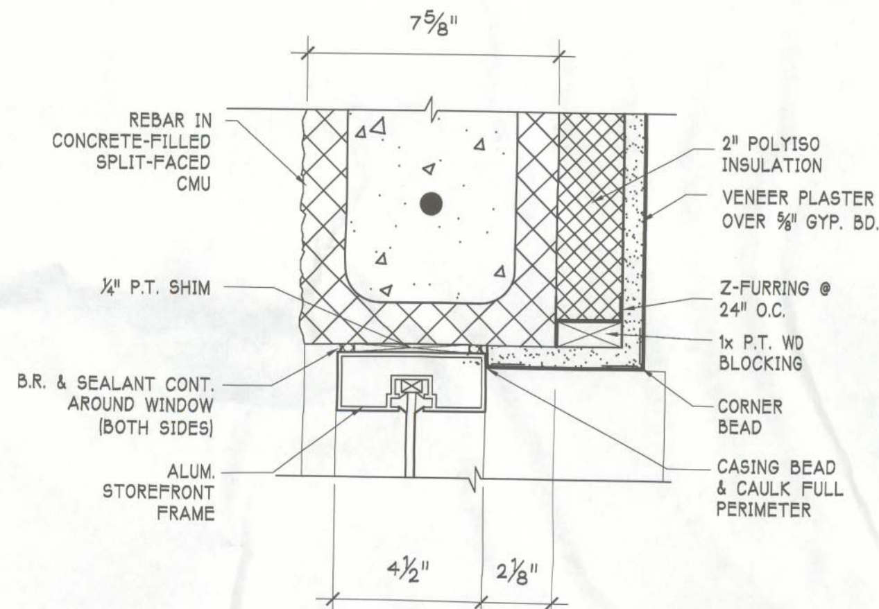
WINDOW JAMB / CMU WALL
