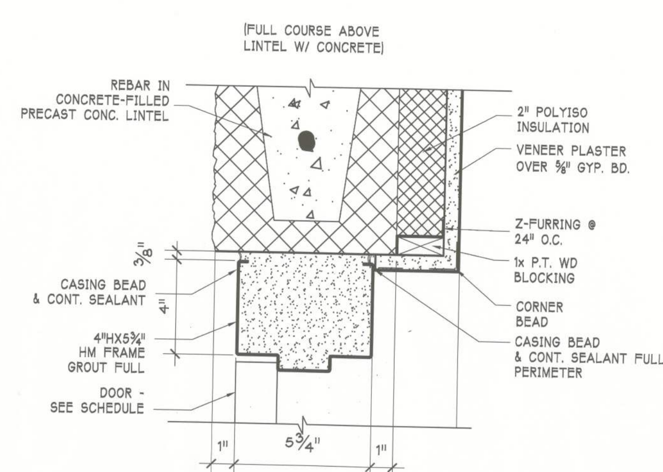
EXT. DOOR HEAD HM FRAME/CMU WALL
