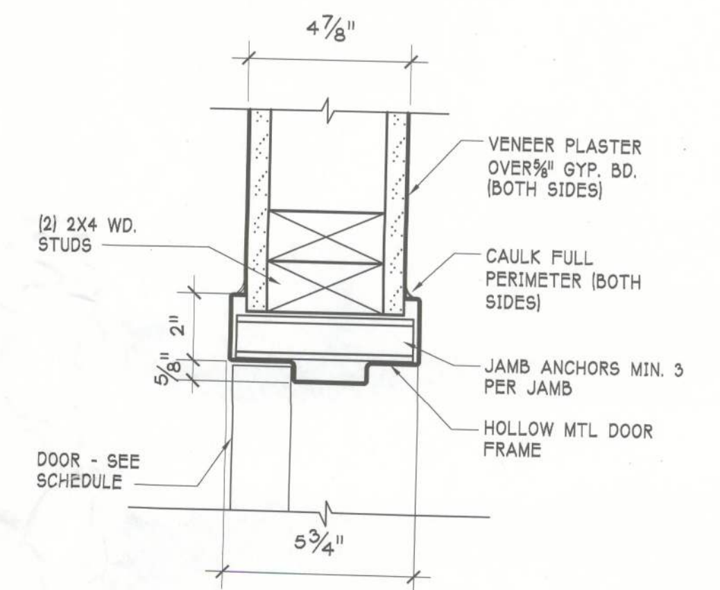
TYPICAL INT. DOOR JAMB HM FRAME/MTL. STUD WALL
