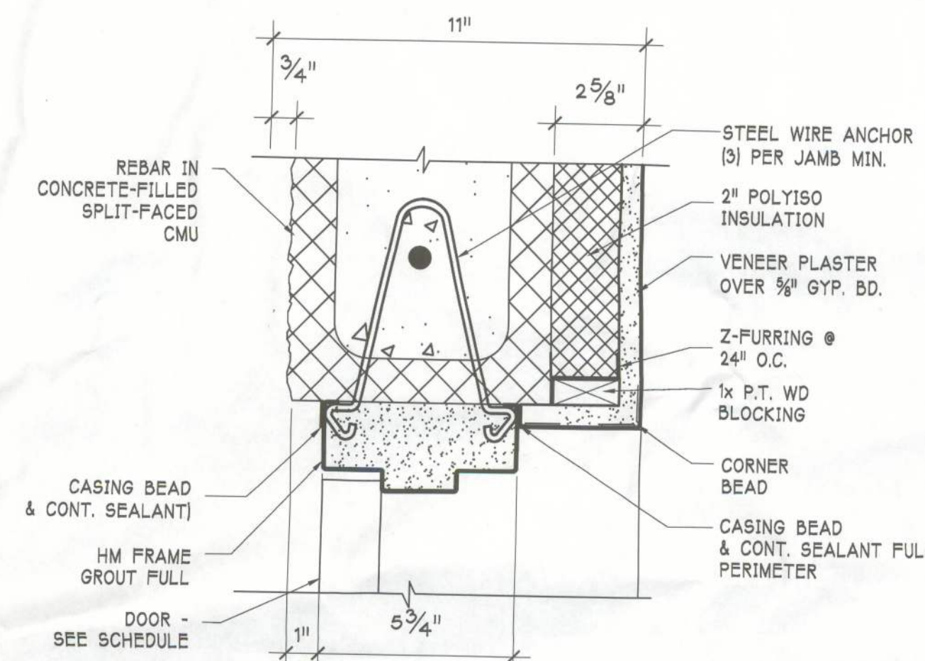
EXT. DOOR JAMB HM FRAME/CMU WALL
