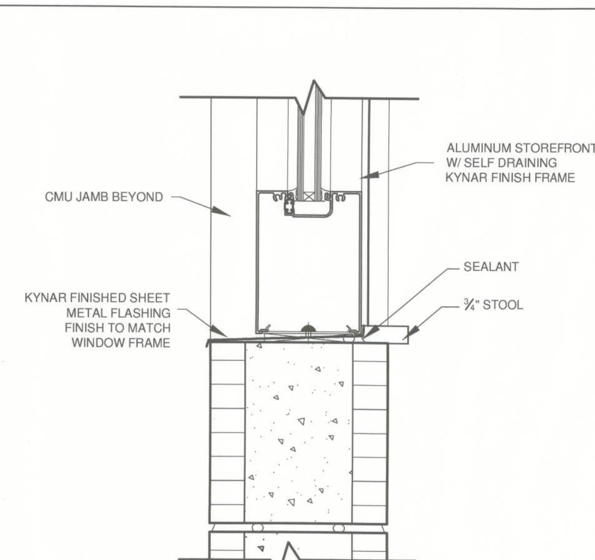
3 A1.4 WINDOW SILL DETAIL SCALE: 3" = 1'-0"
