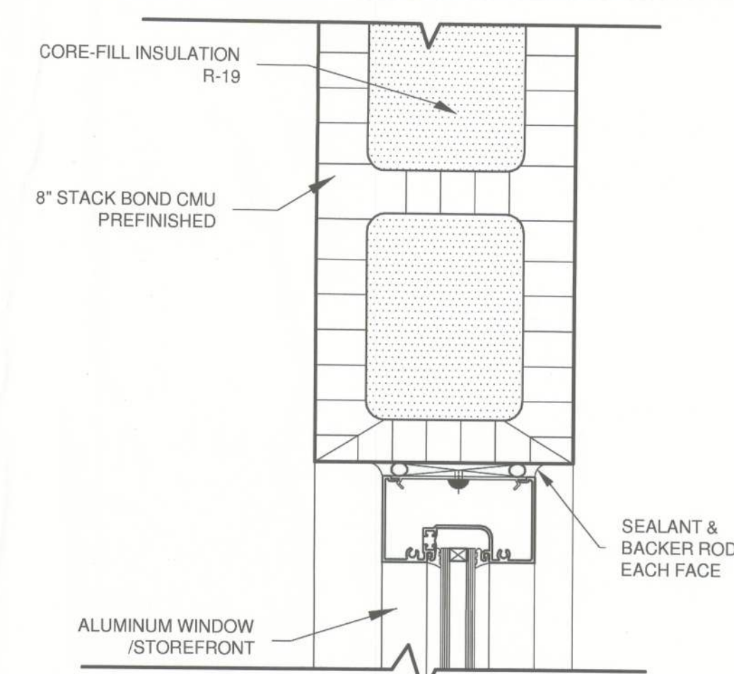
4 A1.4 WINDOW JAMB DETAIL SCALE: 3" = 1'-0"
