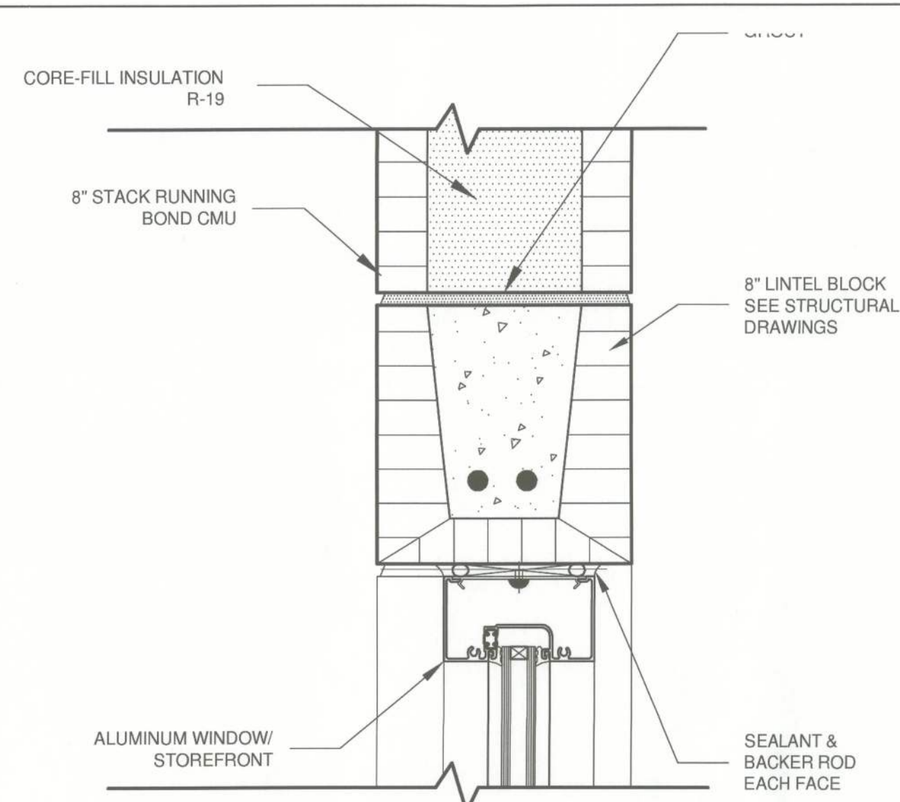
1 A1.4 WINDOW HEAD DETAIL SCALE: 3" = 1'-0"
