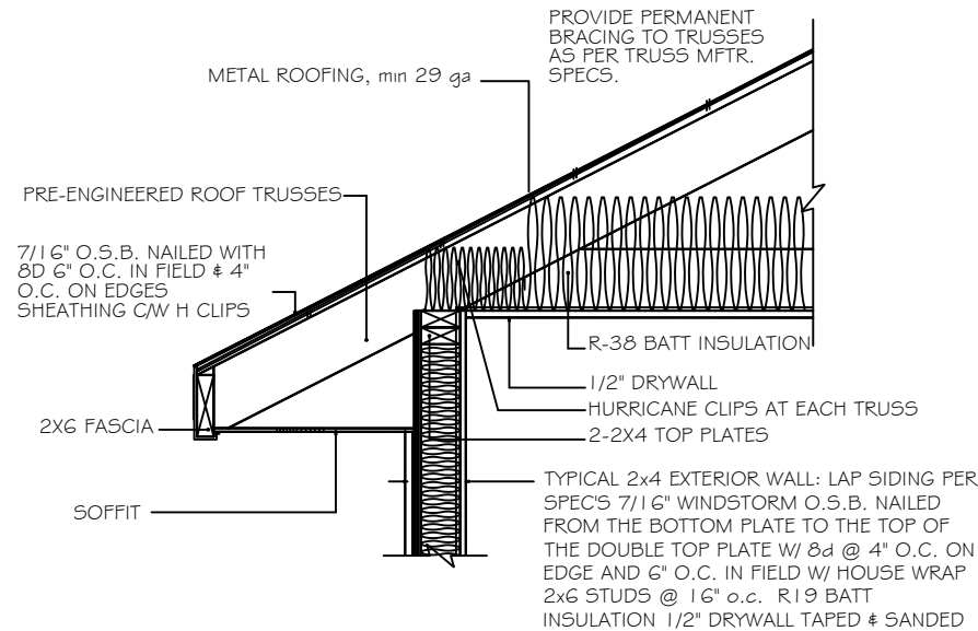
4" STUD EAVE
