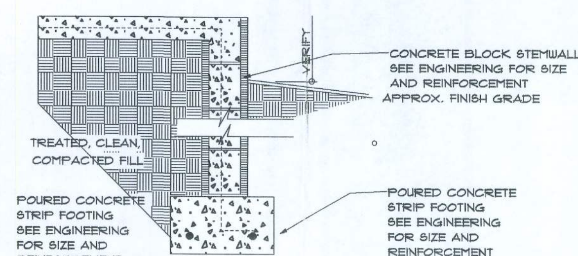
TYPICAL FTG. N.T.S.
