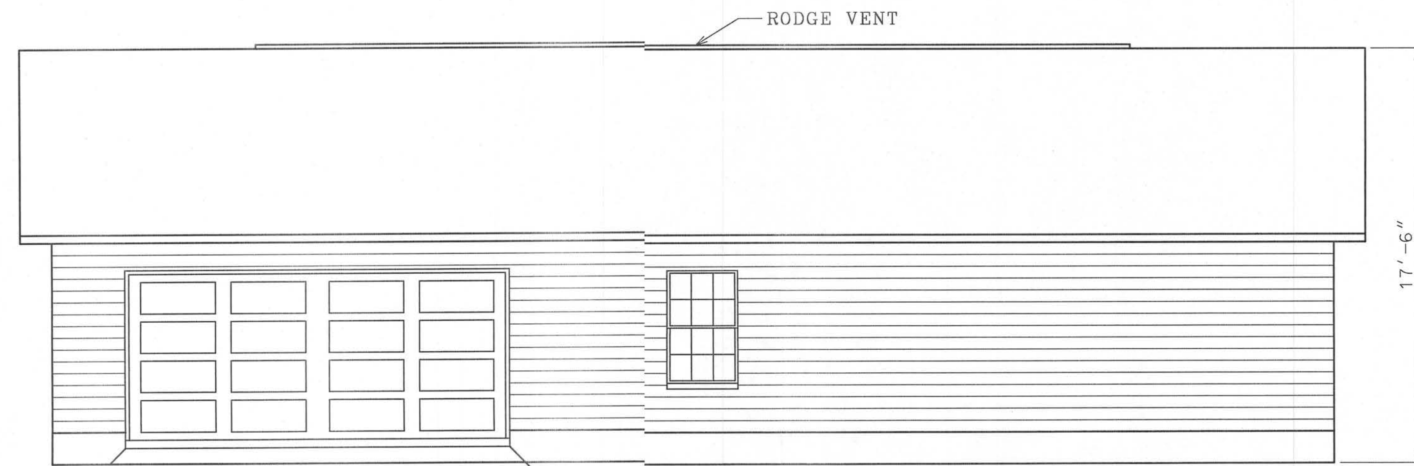
RIGHT ELEVATION
