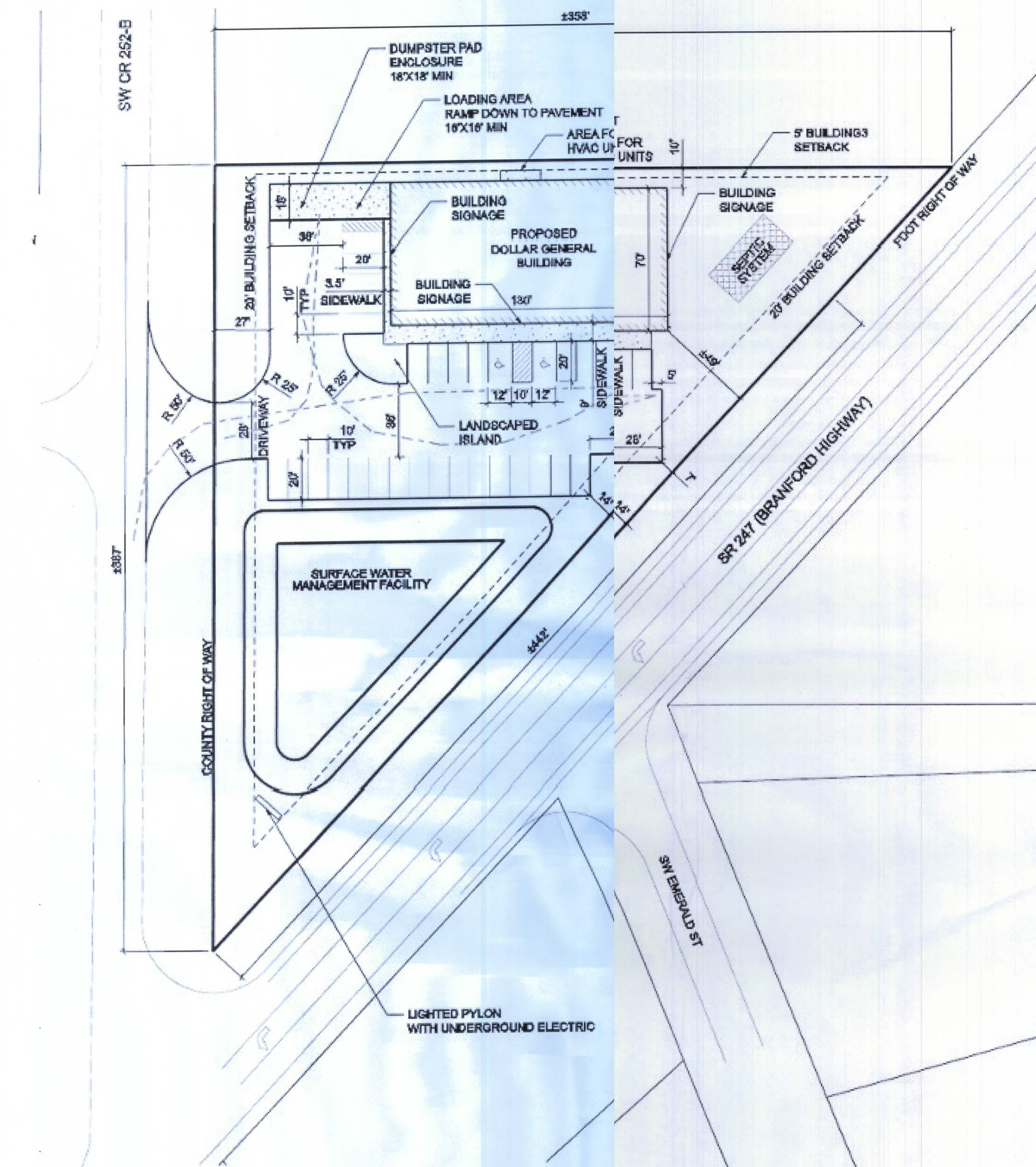
1 SITE PLAN OPTION "C" 1.C N.T.S.
