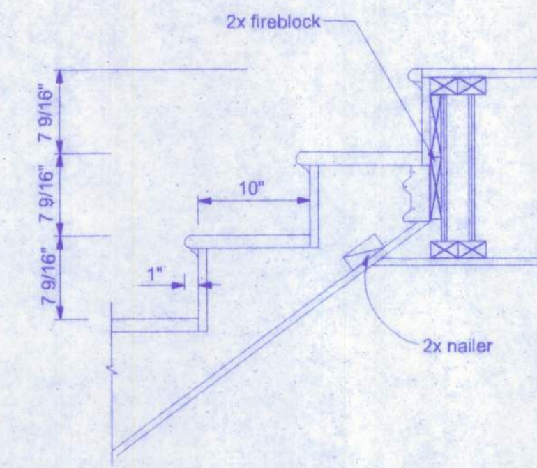
1 HEADER SECTION SCALE: 1" = 1'-0"
