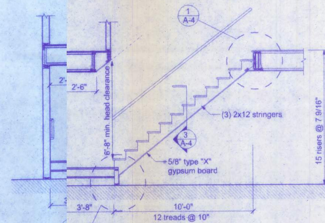
STAIR SECTION SCALE: 1/4" = 1'-0"
