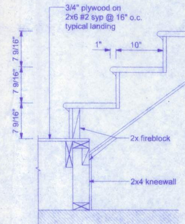
2 BASE SECTION SCALE: 1" = 1'-0"
