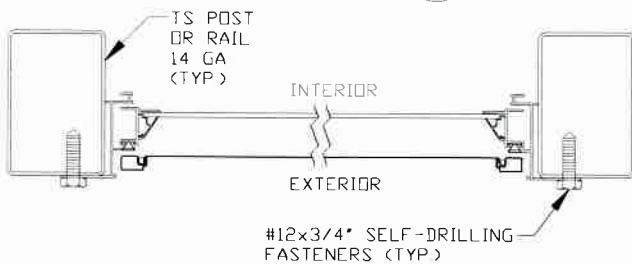
SECTION SCALE: 3\"/>
