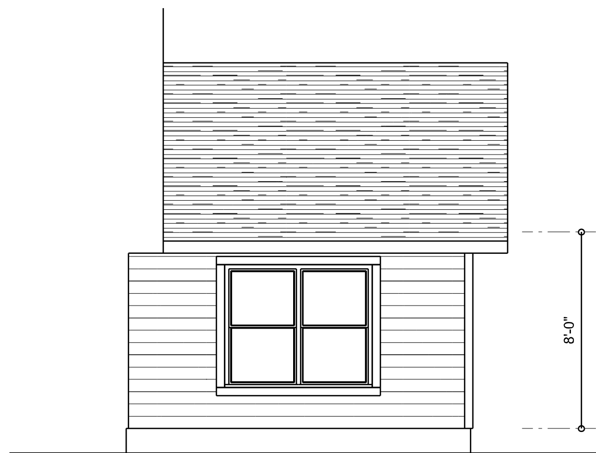
LEFT ELEVATION SCALE: 1/4" = 1'-0"
