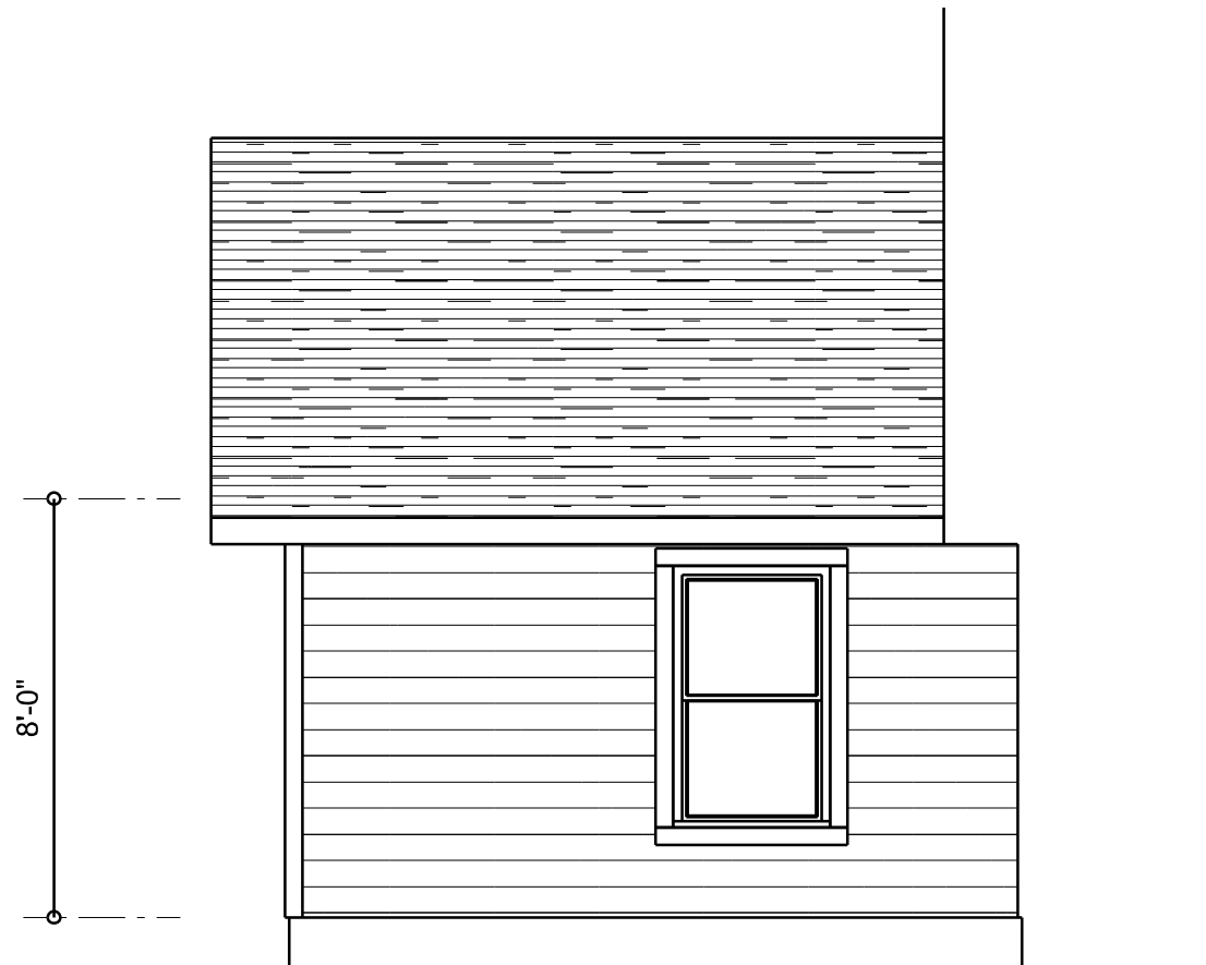
RIGHT ELEVATION SCALE: 1/4" = 1'-0"
