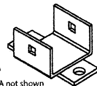
Part # 1101 W-CPCA not shown
