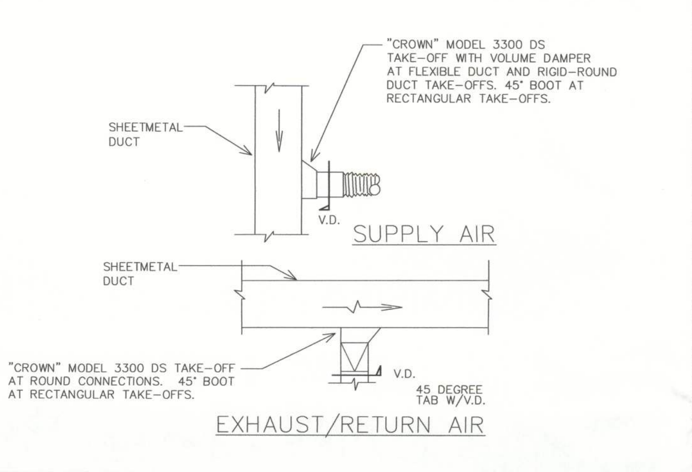
AIR DUCT DETAILS DET 6 M3
