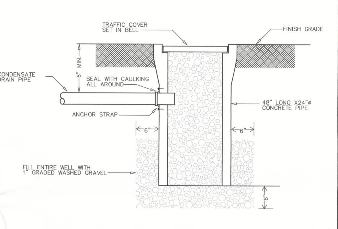
DRYWELL DETAIL DET 7 M3
