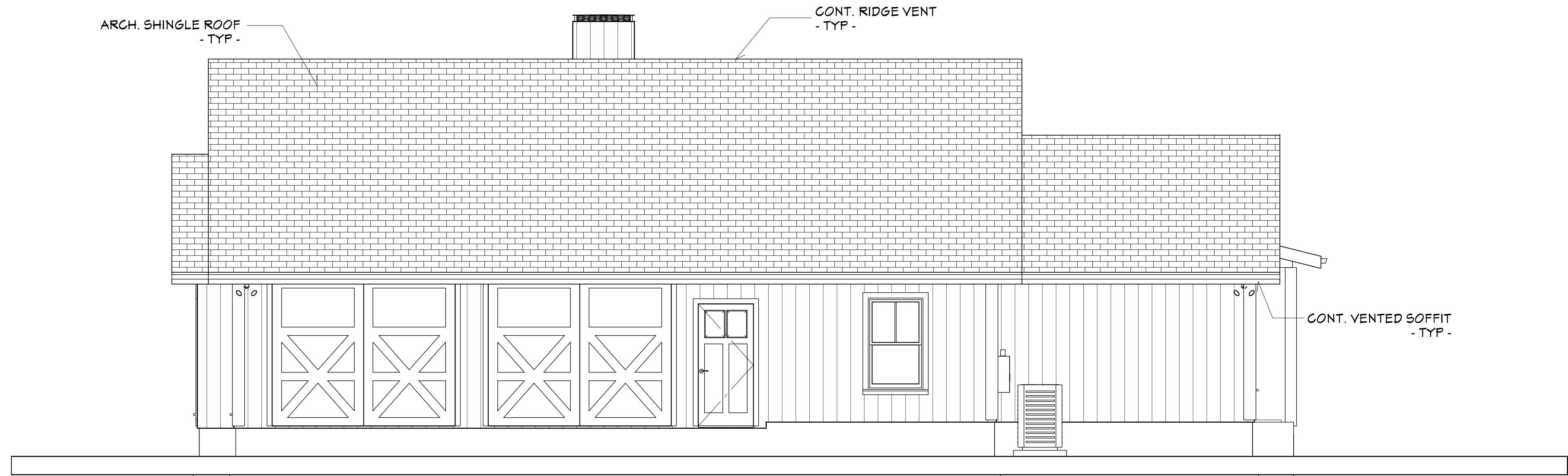
Right Elevation
