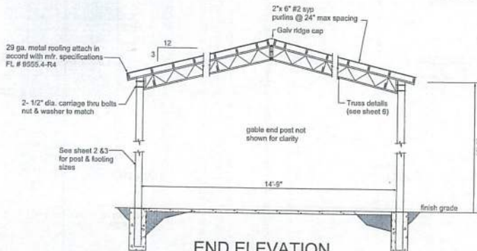
END ELEVATION
