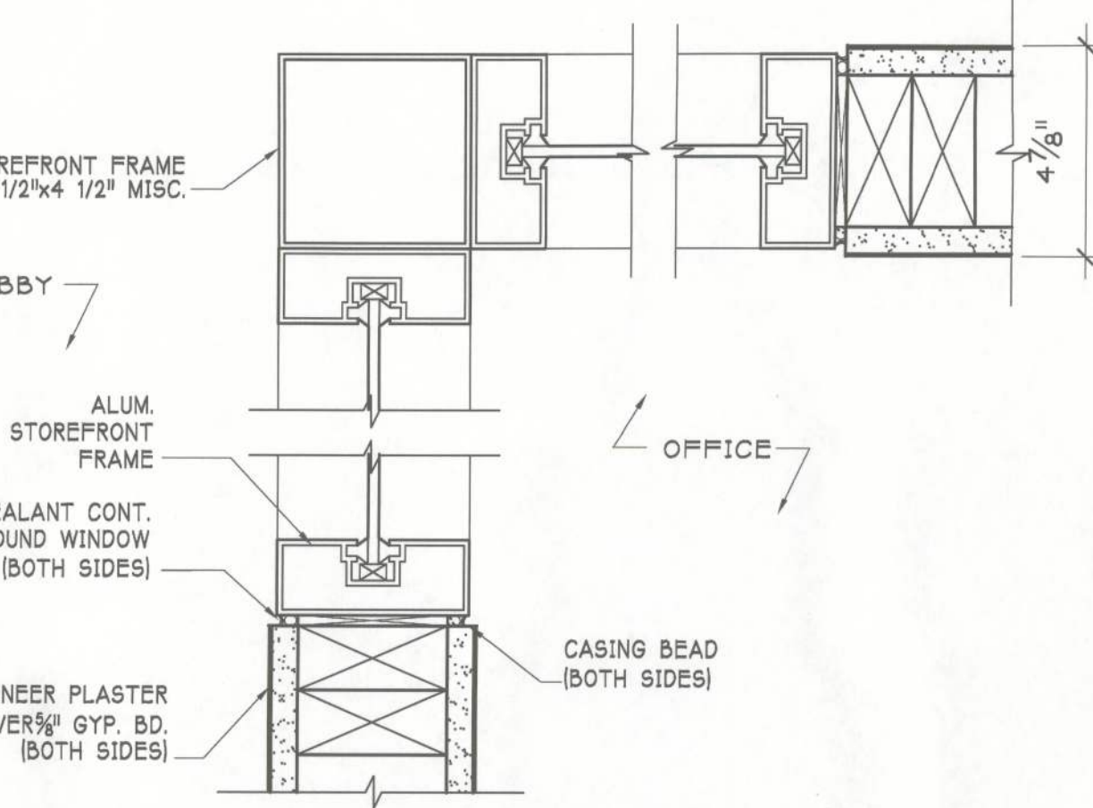
CORNER JAMB OF ALUM STOREFRONT SCALE: 3" = 1'-0"
