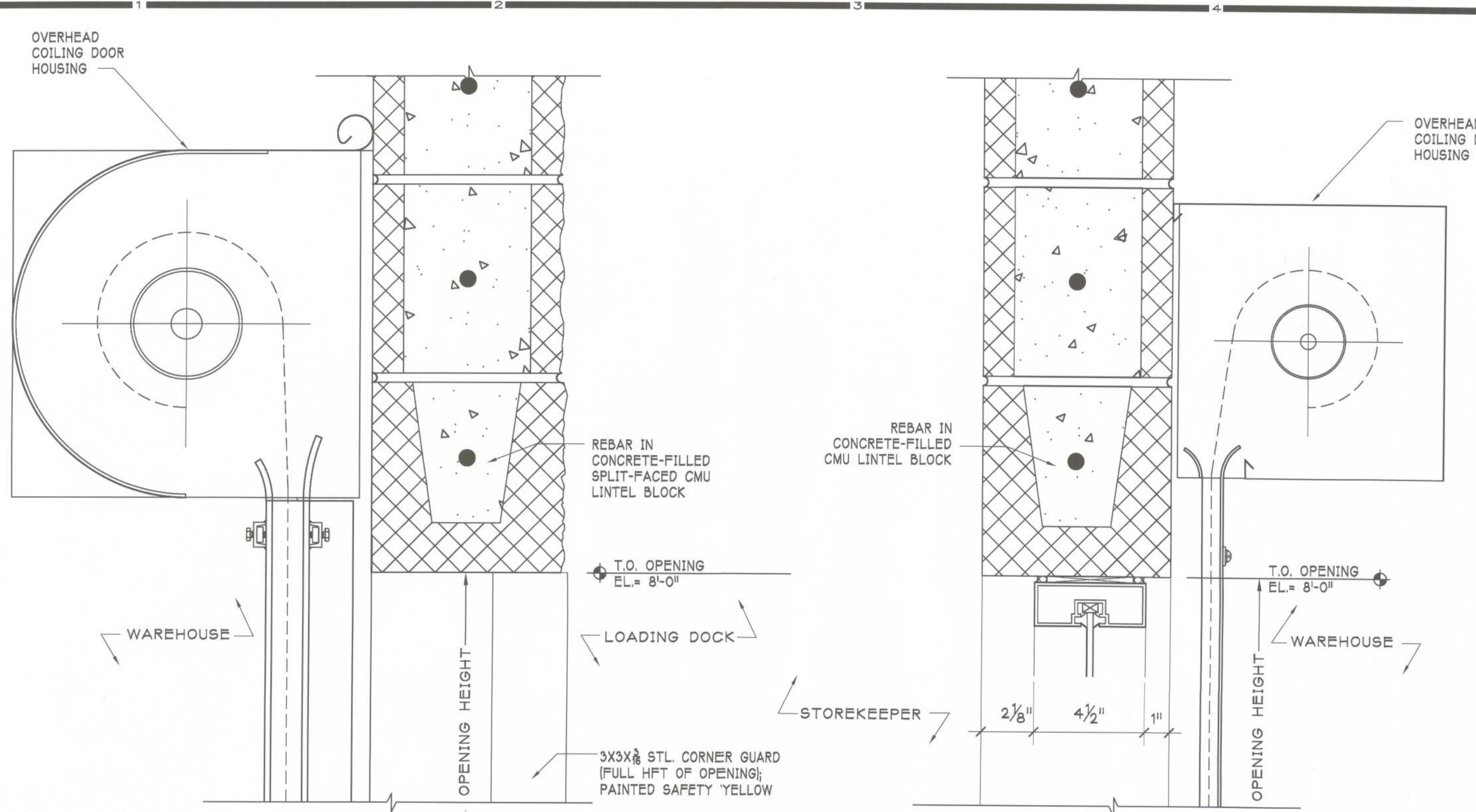
HEAD / COILING DOOR SCALE: 3" = 1'-0"
