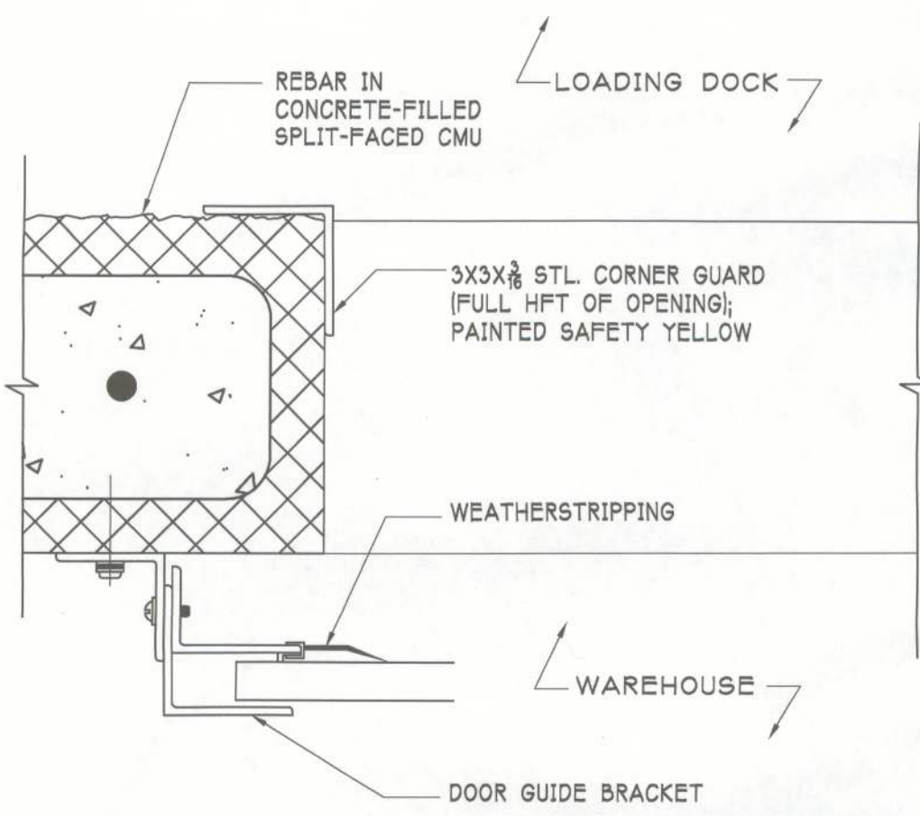
JAMB / COILING DOOR SCALE: 3" = 1'-0"
