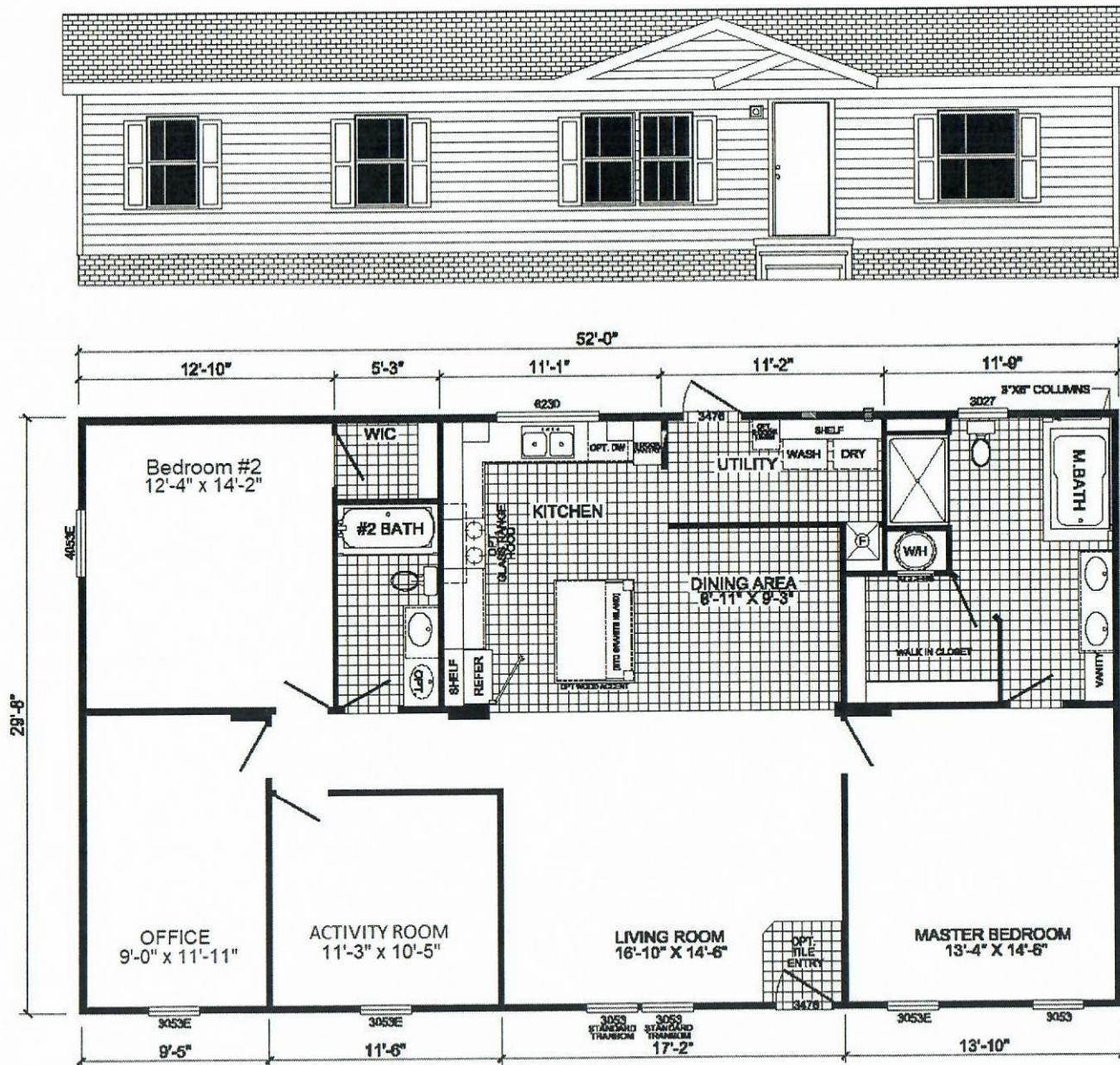
OPTIONAL MASTER BATH
