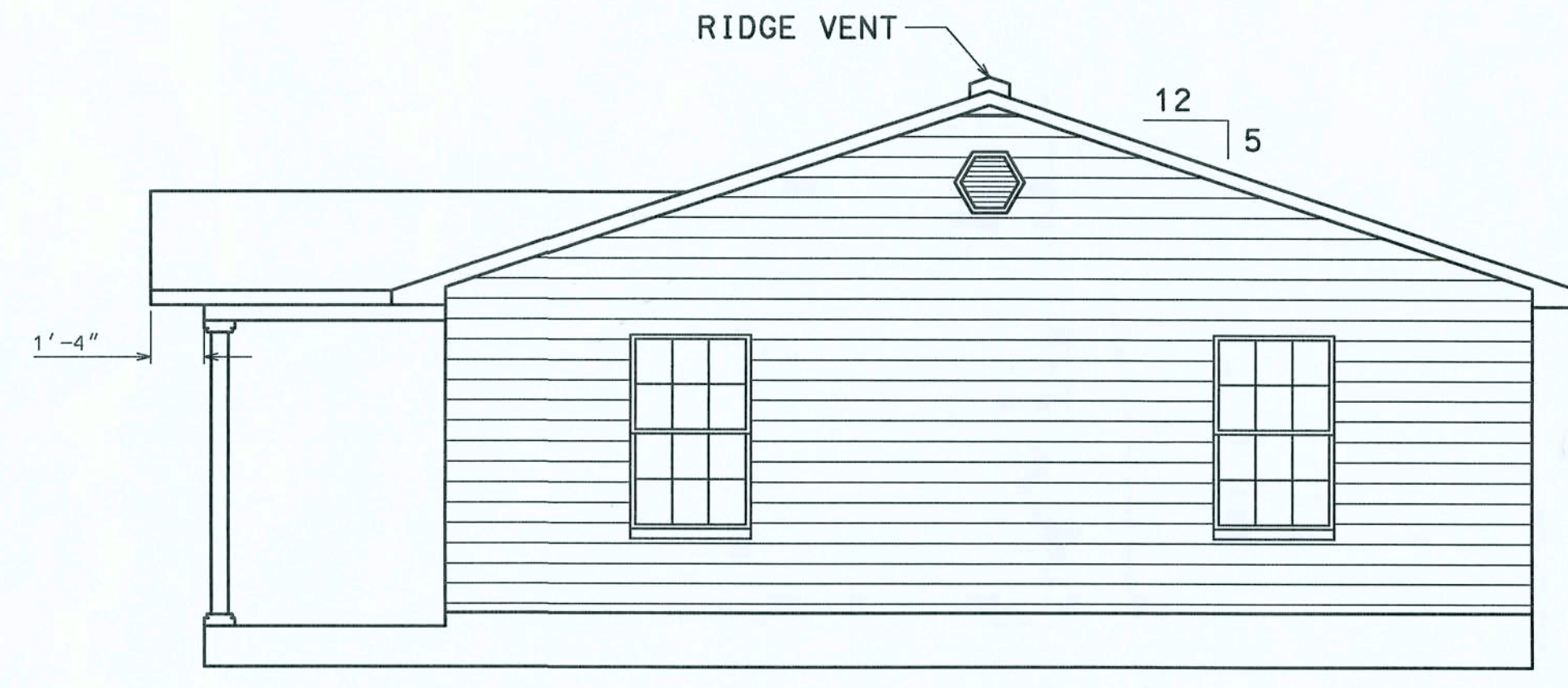
RIGHT ELEVATION
