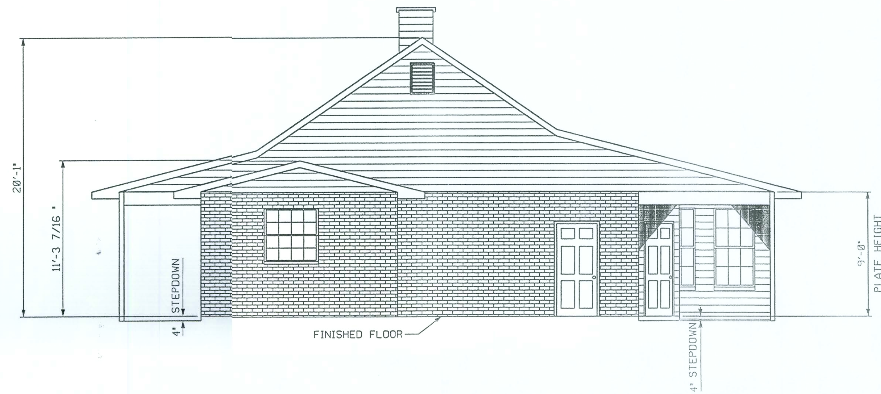
RIGHT ELEVATION
