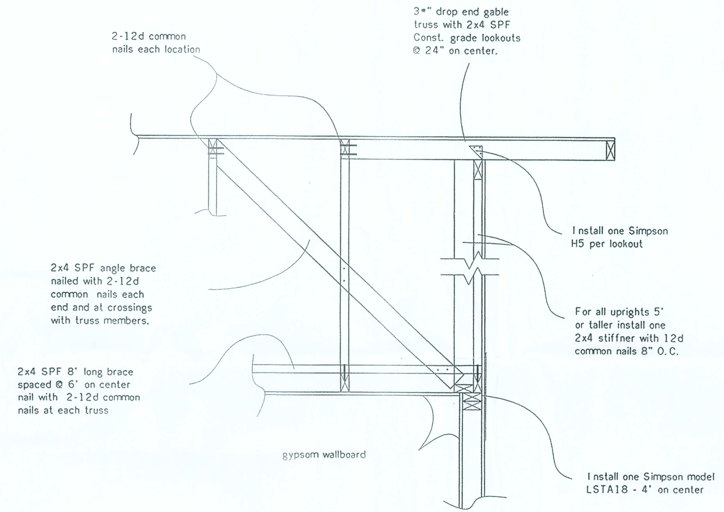
GABLE END BRACING DETAIL (N.T.S.)
