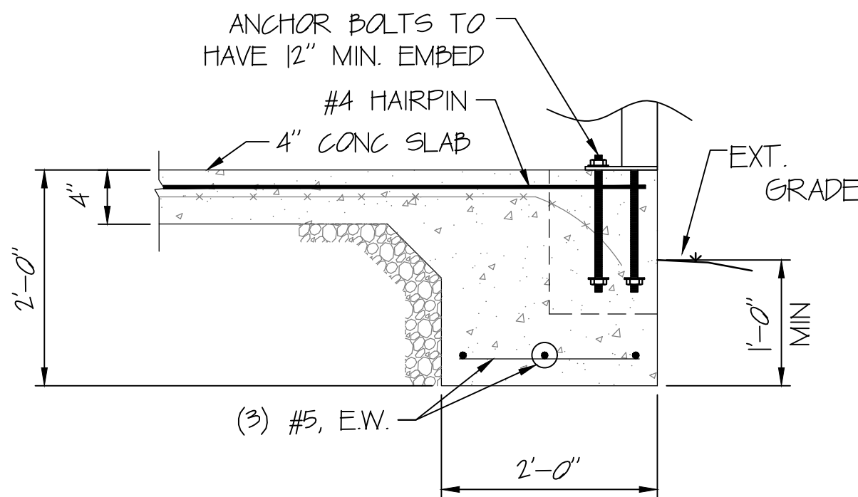
SECTION 2 N.T.S.
