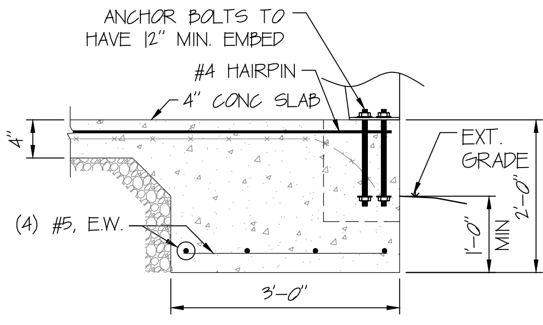
SECTION 3 N.T.S.
