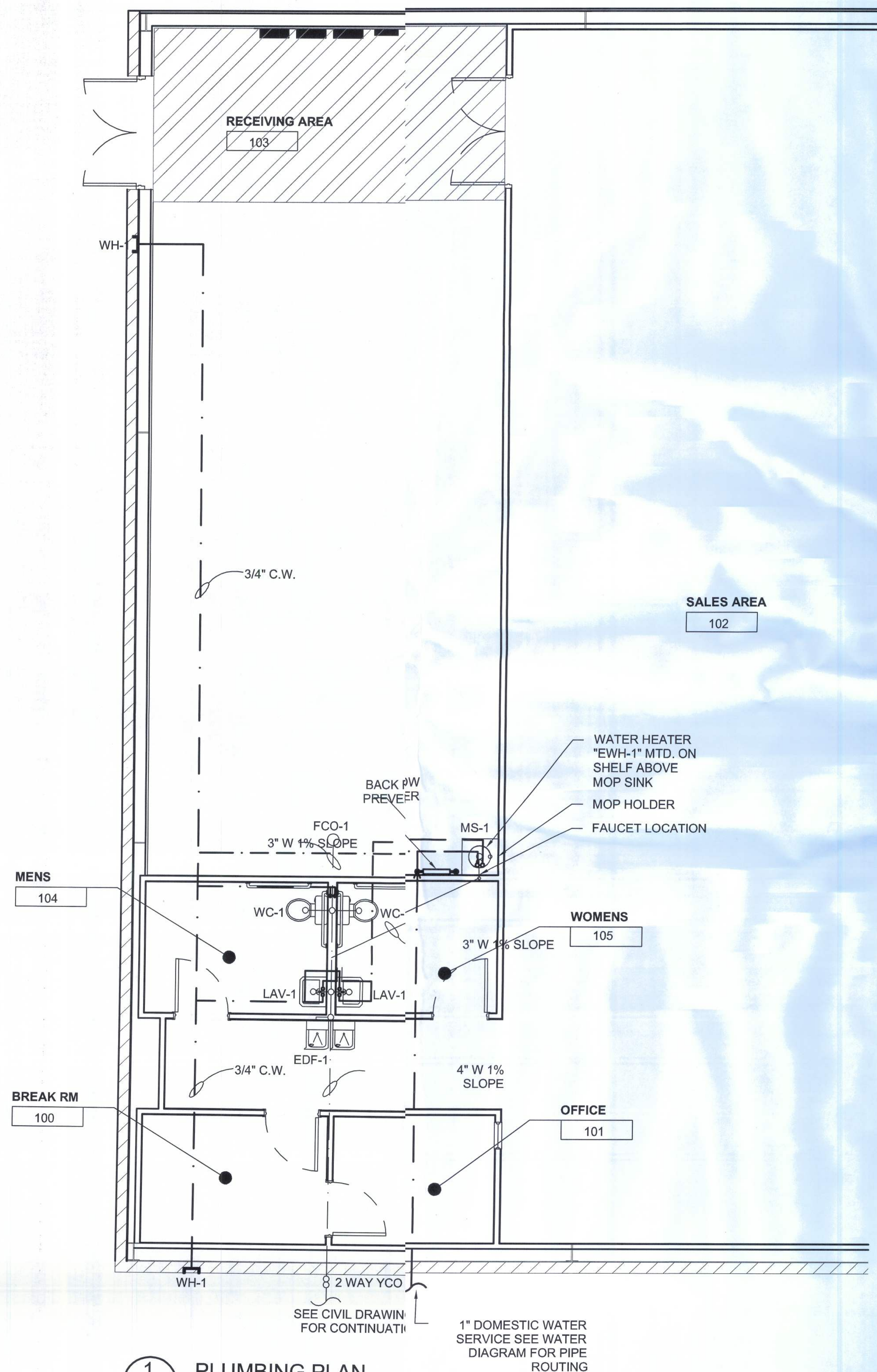
1 PLUMBING PLAN P1.C SCALE: 1/8" = 1'-0"
