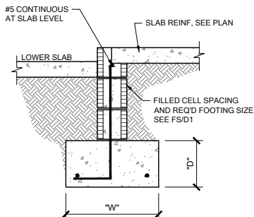
FS03 EXTERIOR BEARING SCALE: 3/4" = 1'-0" @ 22x34 SCALE: 3/8" = 1'-0" @ 11x17
