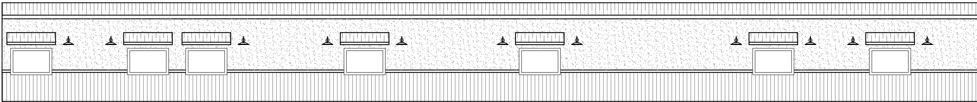
LEFT ELEVATION SCALE: 1/8" = 1'
