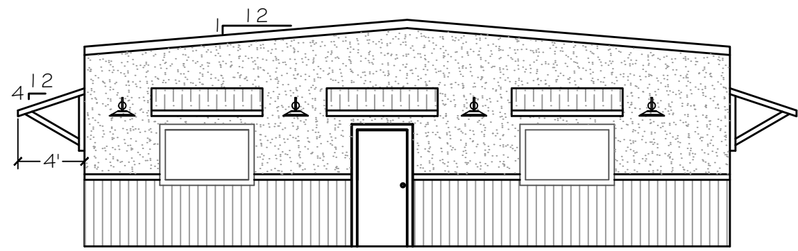
FRONT ELEVATION SCALE: 1/8" = 1'
