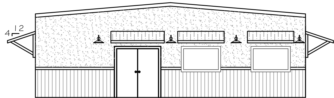
REAR ELEVATION SCALE: 1/8" = 1'
