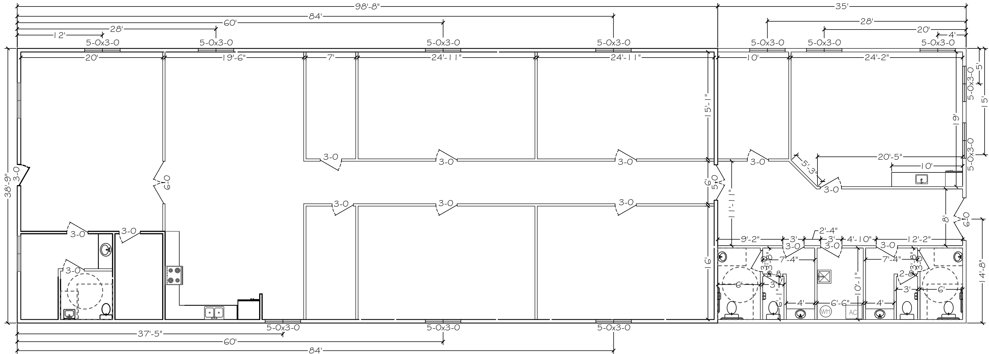
FLOOR PLAN SCALE: 1/8" = 1'
