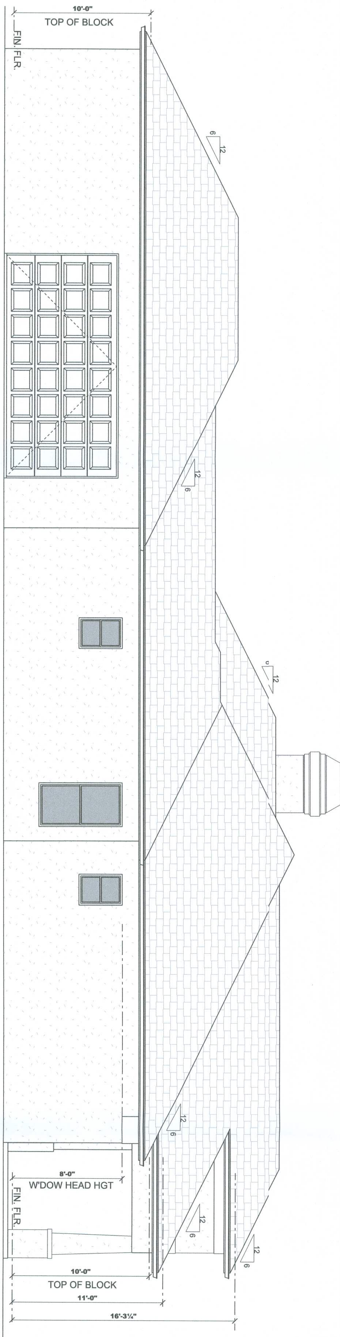
LEFT ELEVATION SCALE: 1/4"=1'-0"
