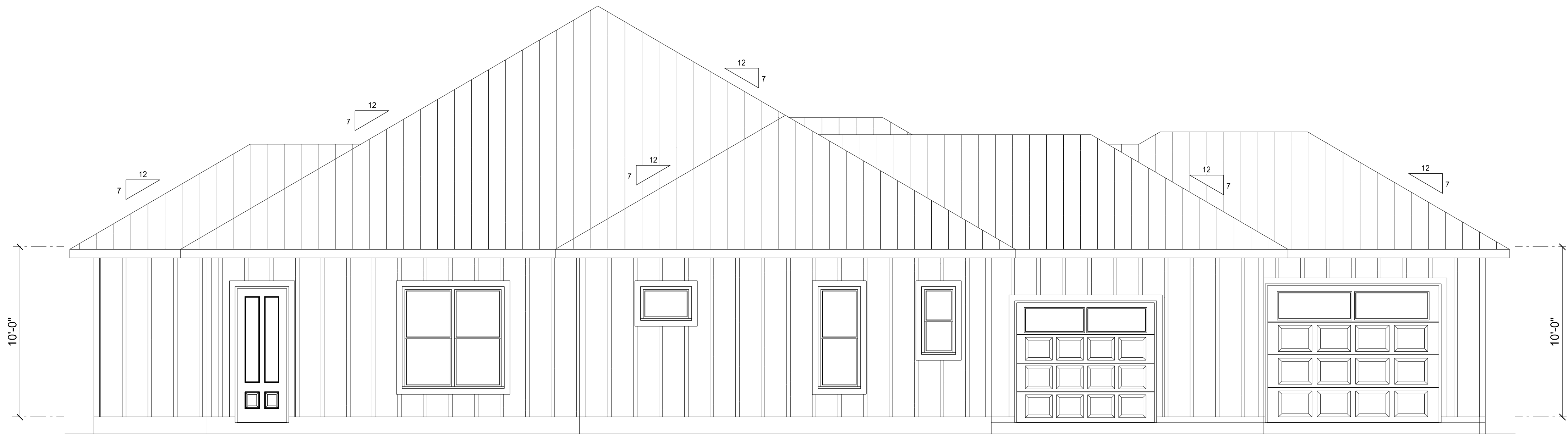
LEFT ELEVATION SCALE: 1/4" = 1'-0"
