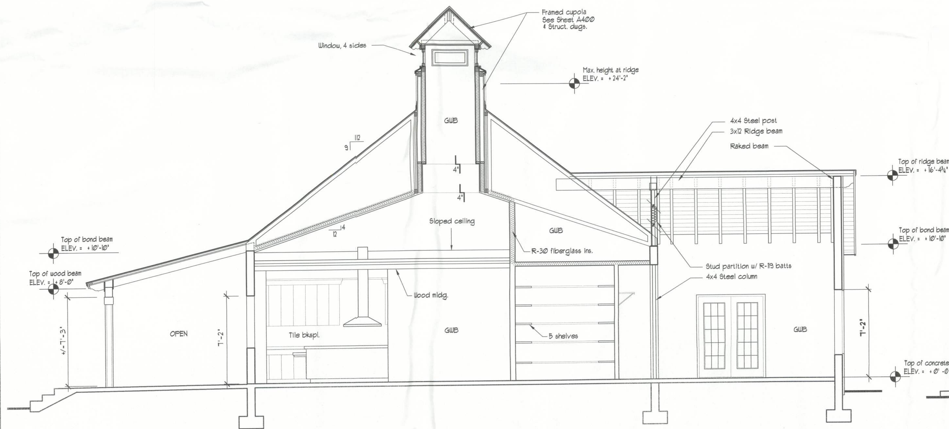
SECTION C scale: 1/4" = 1'-0"
