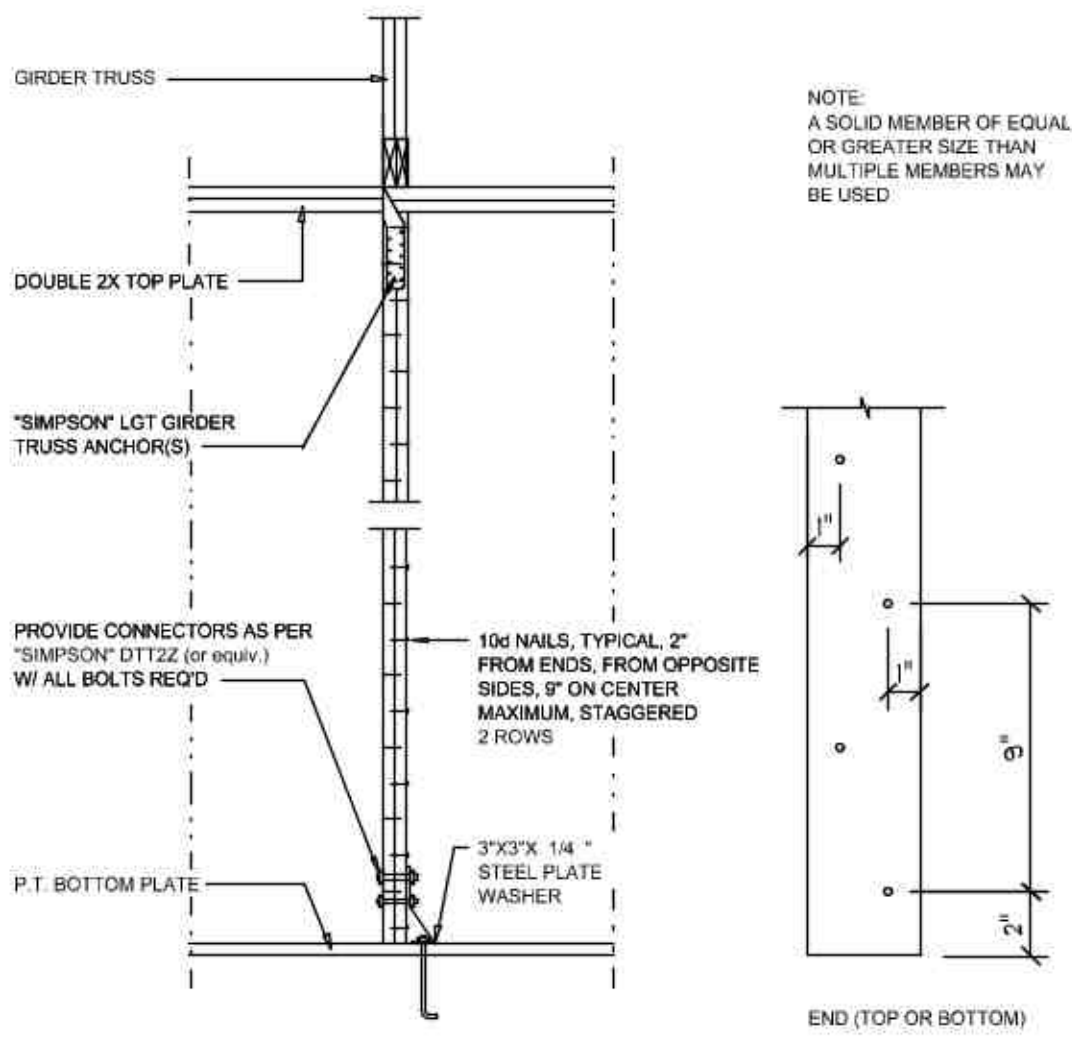
Girdler Truss Column DET.
